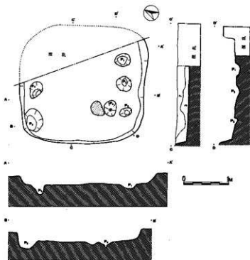
第21図 戸神遺跡第2号住居址平面実測図
