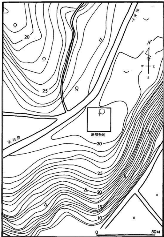
第7圖 鐵道遺跡全測圖
