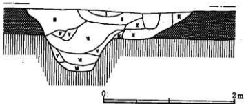
第6図 2号遺構実測図
