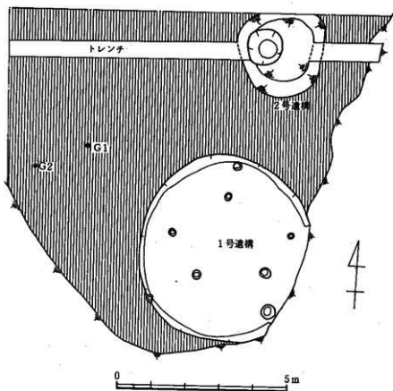
第3図 遺跡全測図
