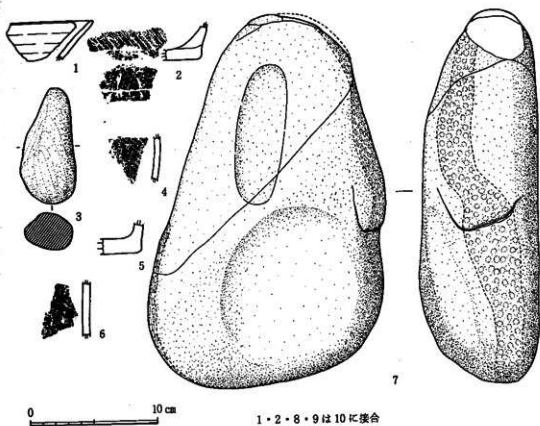
第5図 1号遺構出土遺物実測図
