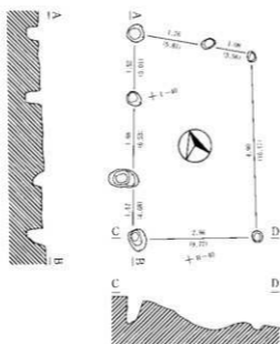
第32号掘立柱建物跡
