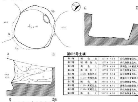
第362図 第613・614・615号土壤
