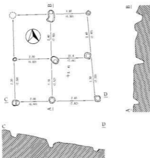
第35号掘立柱建物跡
