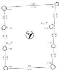
第8号掘立柱建物跡
