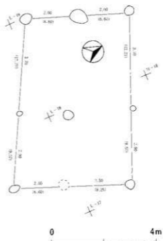
第15号掘立柱建物跡 (模式図)
