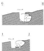
第310号住居跡カマド
