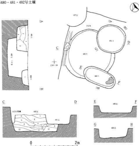
第306图 第479·480·481·482号土壤
