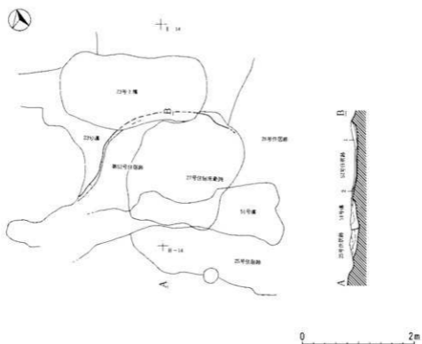
第52号豎穴住居跡
