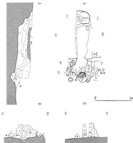
第310号住居跡カマド
