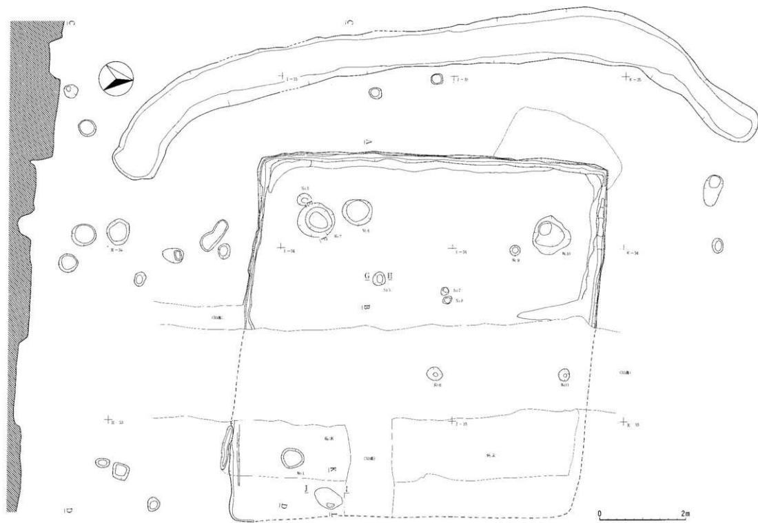
第20図 第33号竪穴住居跡(1)
