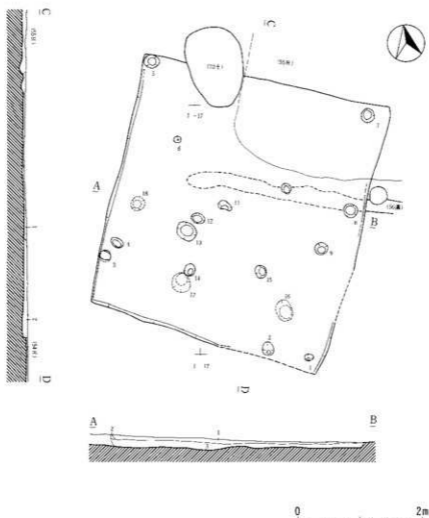
第53号竖穴住居跡
