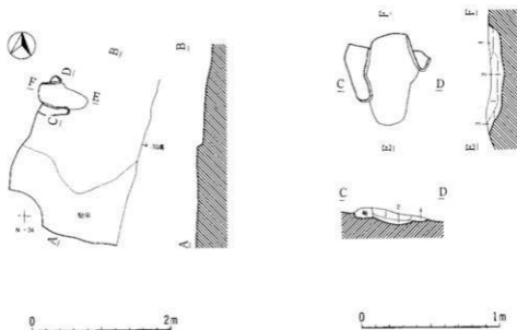
第48号住居跡カマド
