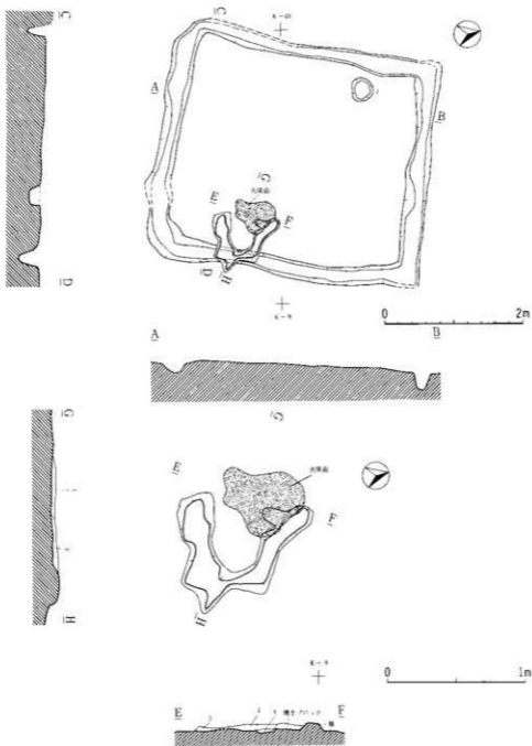
第128号住居跡カマド
