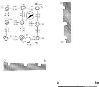
第7号掘立柱建物跡
