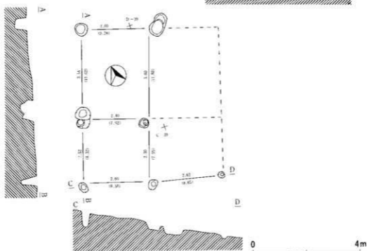
第39号掘立柱建物跡
