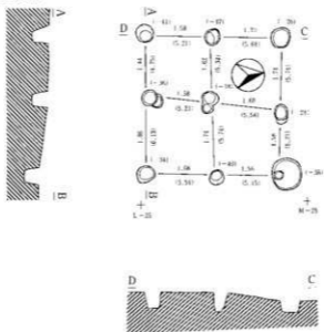
第6号掘立柱建物跡
