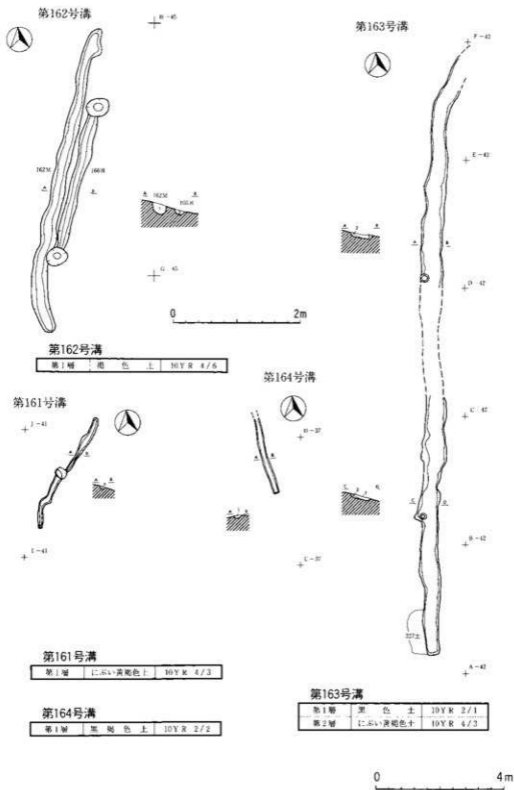
第463図 第161・162・163・164号溝
