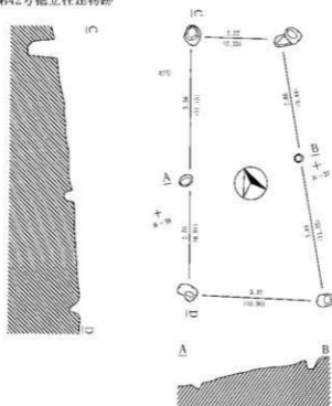
第43号掘立柱建物跡
