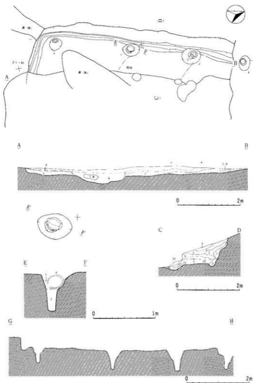
第154图 第316号窑穴住居跡
