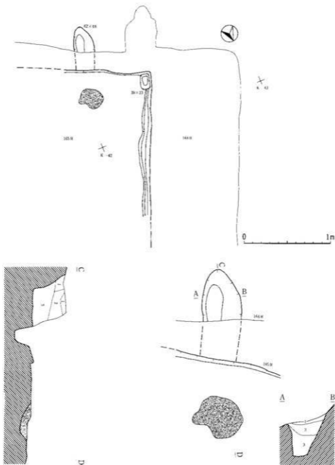
第165号住居跡カマド
