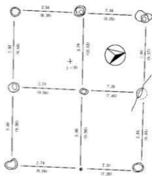
第27号掘立柱建物跡
