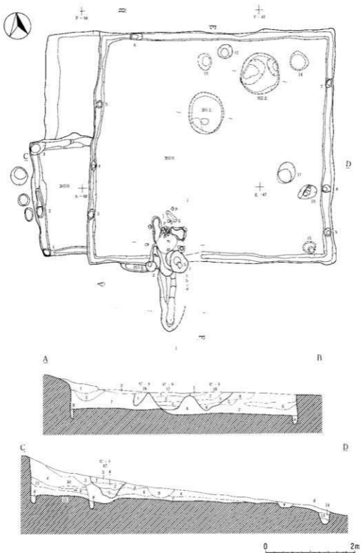
第138图 第302·303号竖穴住居跡
