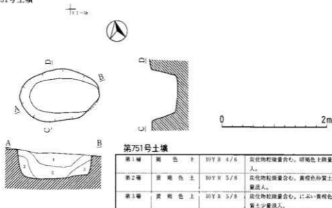
第415図 第750・751号土壤
