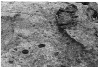
第52号竪穴住居跡、23・51溝
