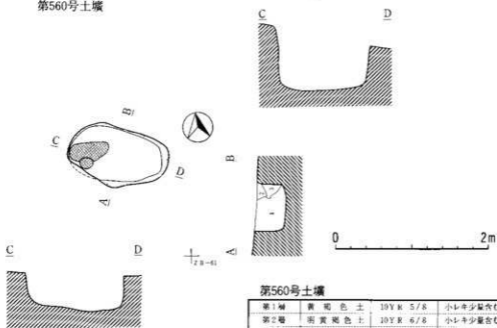
第340図 第558・559・560号土壌
