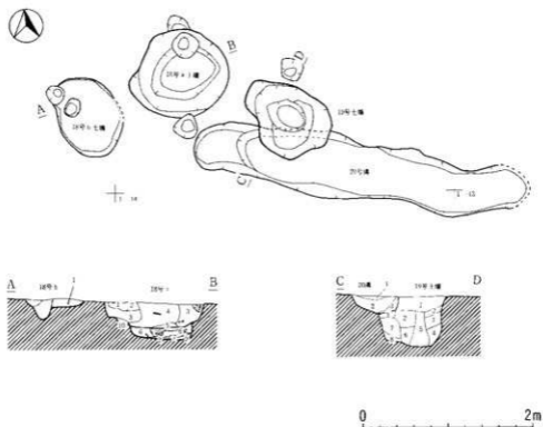
第18 a・18 b・19号土壤・第20号溝
