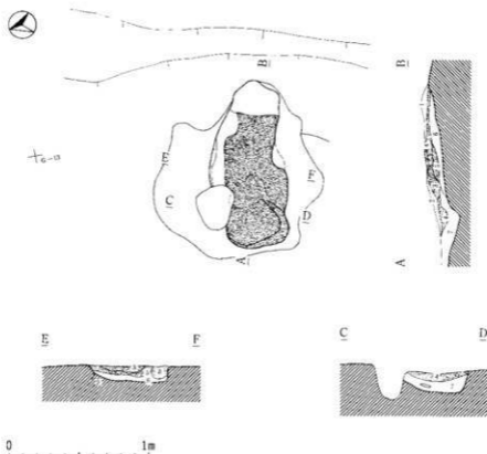
第66号住居跡カマド
