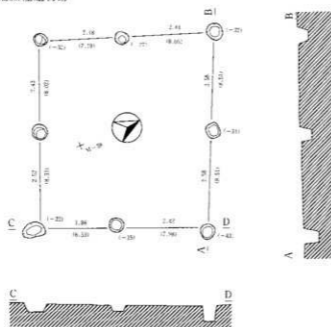
第3号掘立柱建物跡
