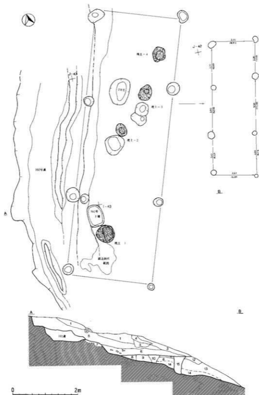
第465图 鑛冶遺構（第30号掘立柱建物跡）- 1
