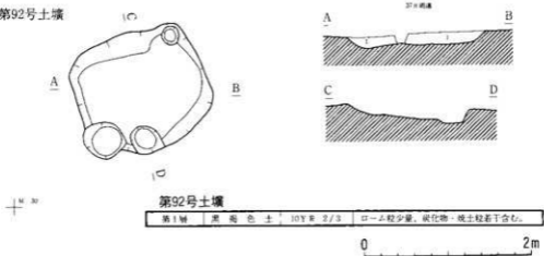
第202図 第87・91・92号土壕
