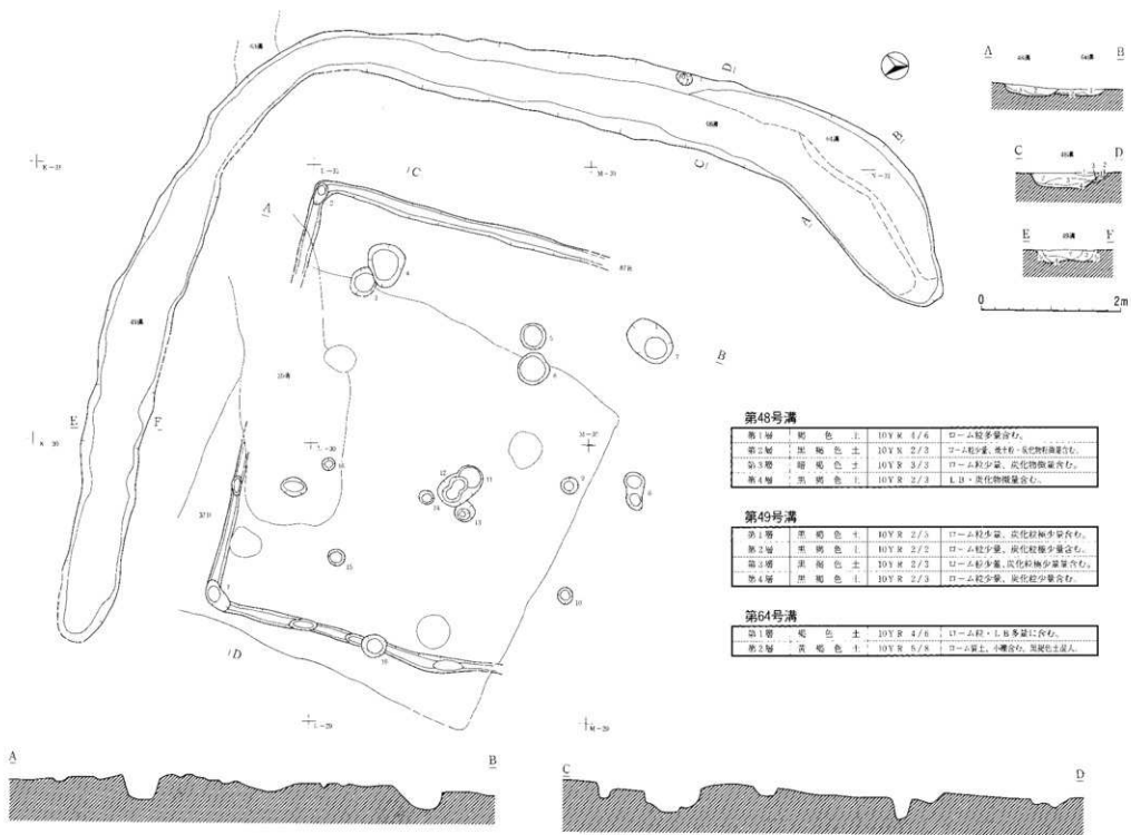
第62図 第87号竪穴住居跡・第48・49・64号溝
