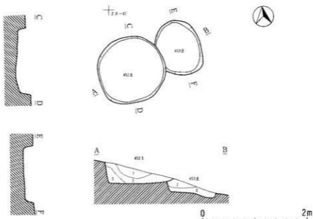
第294図 第451・452・453号土壤
