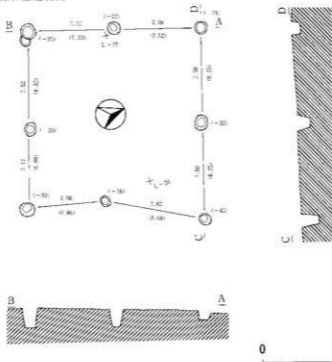
第5号掘立柱建物跡
