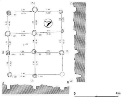
第167图 第20・21号掘立柱建物跡
