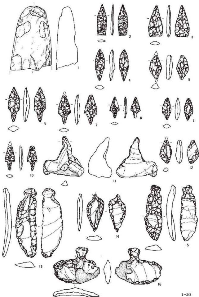
图133 遺構外出土石器(1)
