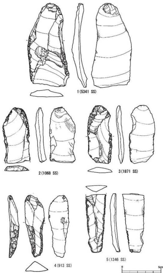
図版21 笹山原No. 27遺跡表探のサイド・スクレイパー Fig. 21 Side-scrapers at the Sasayamahara No. 27 site.
