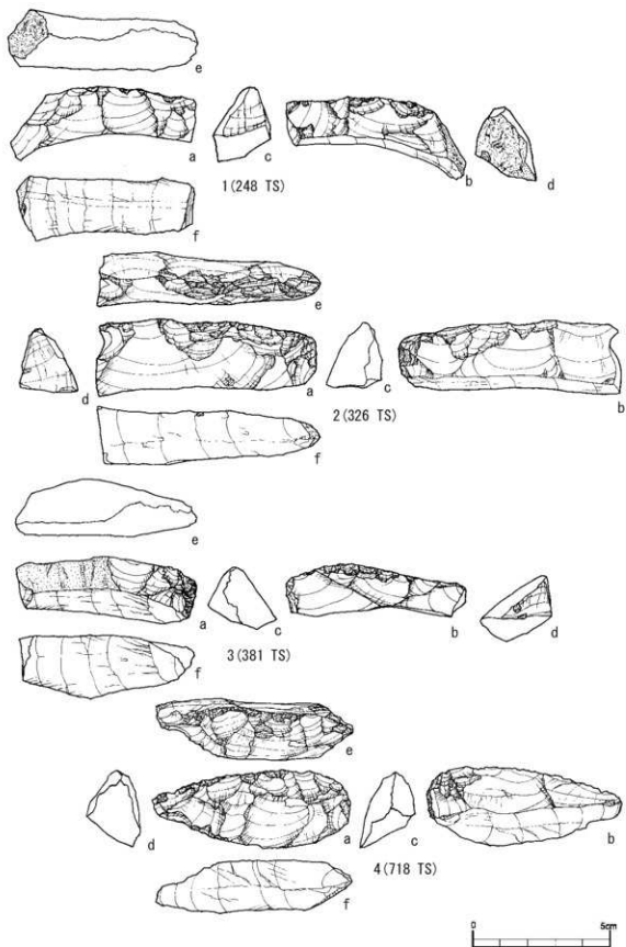
図版10 笹山原No. 27遺跡表採のファーストスボール Fig.10 First spalls at the Sasayamahara No. 27 site.
