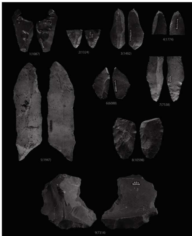
写真図版 19 笹山原 No.27 遺跡出土彫刻刀形石器、尖頭器、調整剥片 Scale=80%
