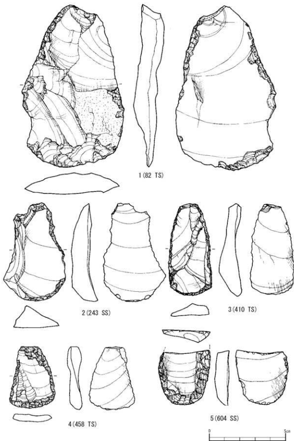
図版19 笹山原No. 27遺跡表採のエンドスクレイパー Fig. 19 End-scrapers at the Sasayamahara No. 27 site.
