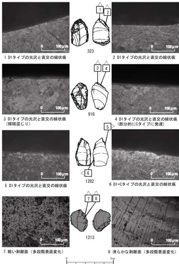
図版26 笹山原No. 27遺跡の彫刻刀形石器の使用痕と表面状態 Fig. 26 Use-wear on burins
