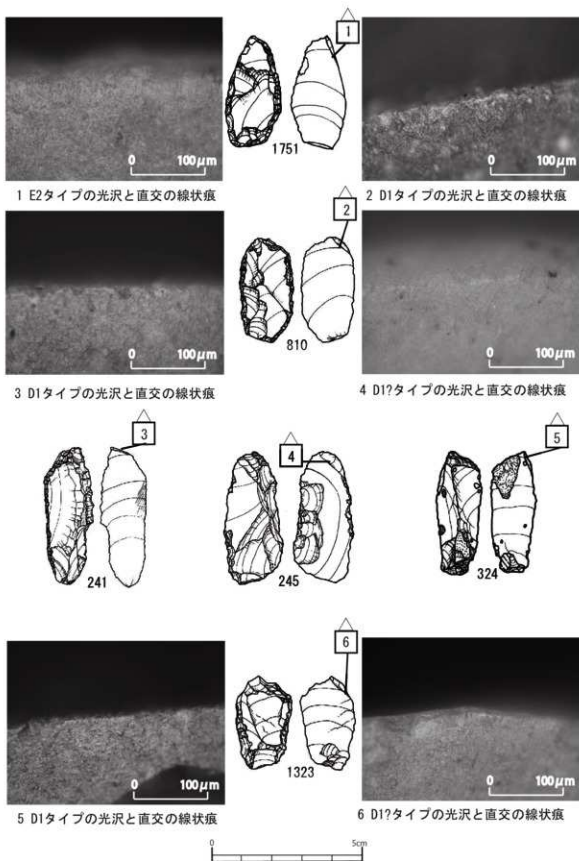
図版27 笹山原No. 27直跡の彫刻刀形石器の使用痕と表面状態 Fig. 27 Use-wear on burins.
