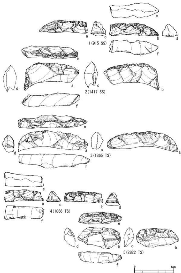
図版11 笹山原No. 27遺跡表採のファーストスポール Fig.11 First spalls at the Sasayamahara No. 27 site.
