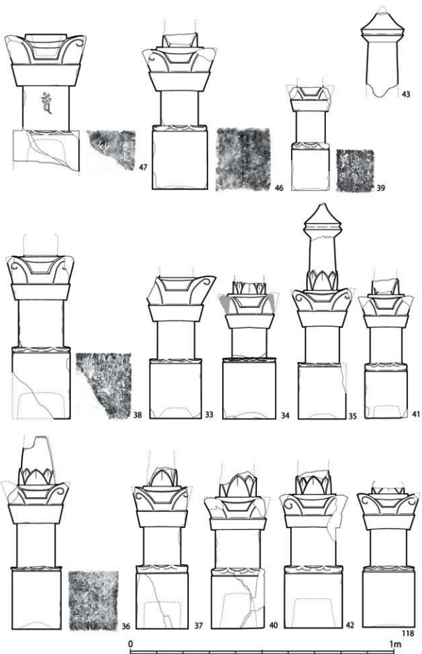
第12図 字基光院東側尾根の石造物実測図1 S=1/10
