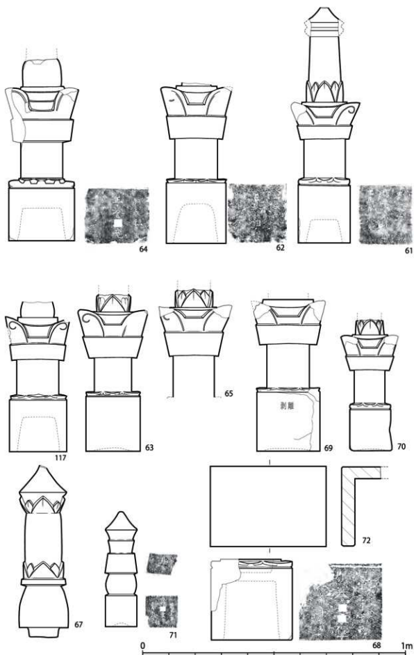
第16図 字基光院西・北側斜面の石造物実測図1 S=1/10
