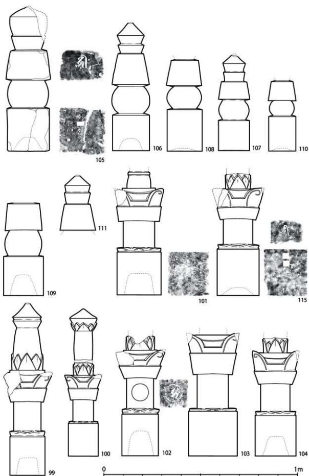
第21図 字基光院南側斜面の石造物実測図 1 S=1/10
