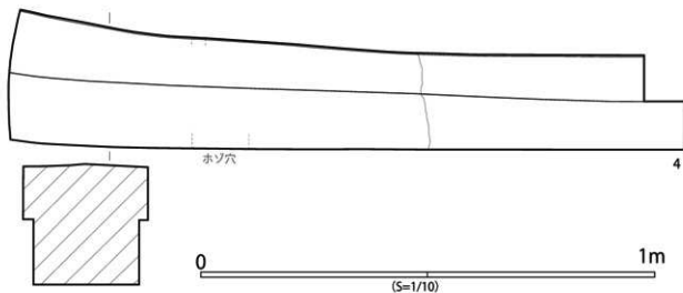
鳥居笠木の全容推定図
