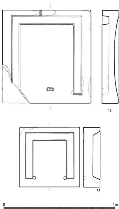
第10図 字基光院尾根頂部の石造物実測図2
