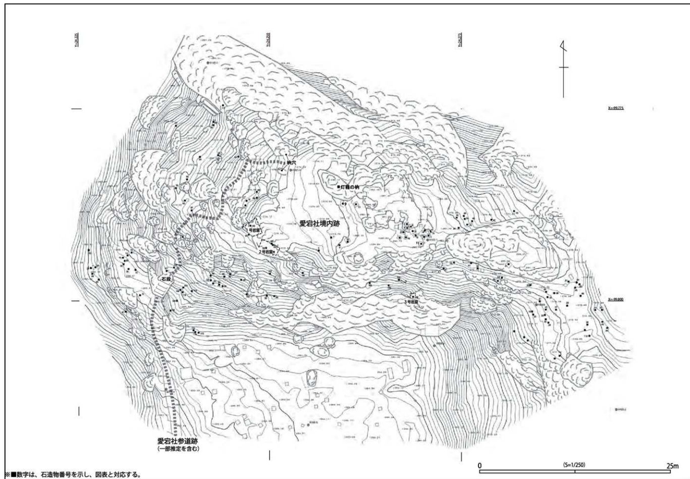
第5図 石見銀山遺跡栃畑谷地区字甚光院墓地周辺図 S=1/250
