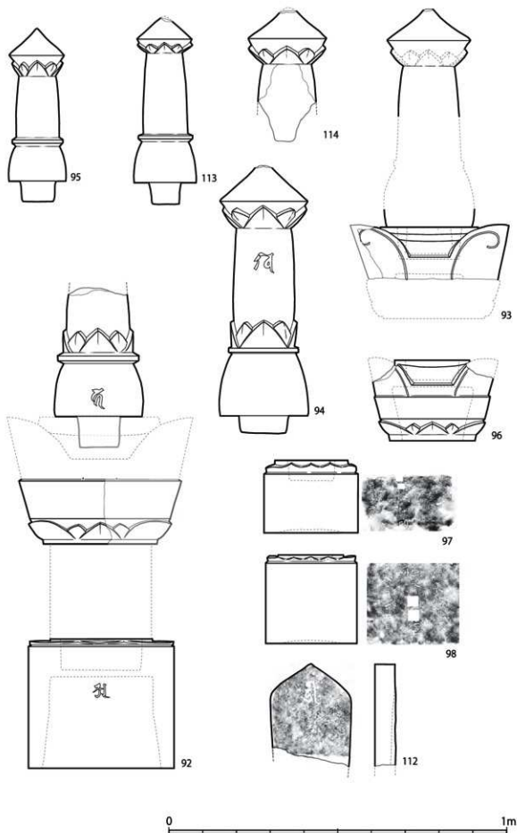
第22図 字基光院南側斜面の石造物実測図 2 S=1/10
