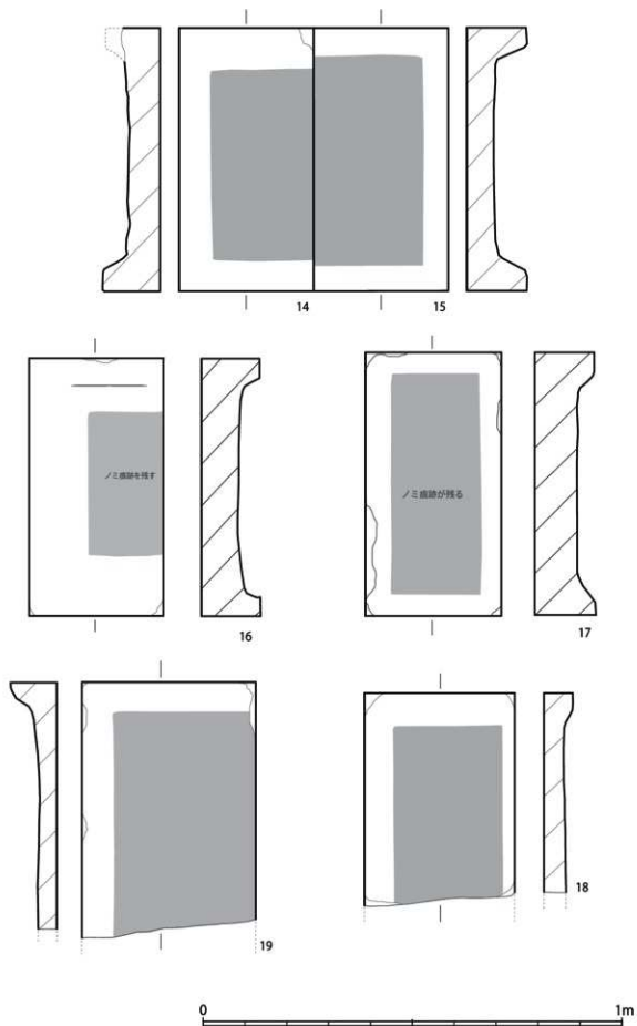
第11図 字基光院尾根頂部の石造物実測図 3 S=1/10
