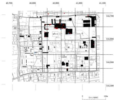
第 34 図 鏡瓦出土位置図 SKM02・03A (S=1/4000)
