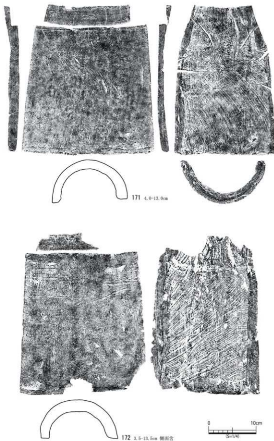
第 59 図 男瓦③ (S=1/4)
