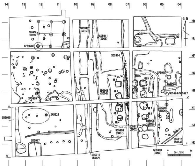
第3図 昭和59年度調査遺構図① (S=1/200)
