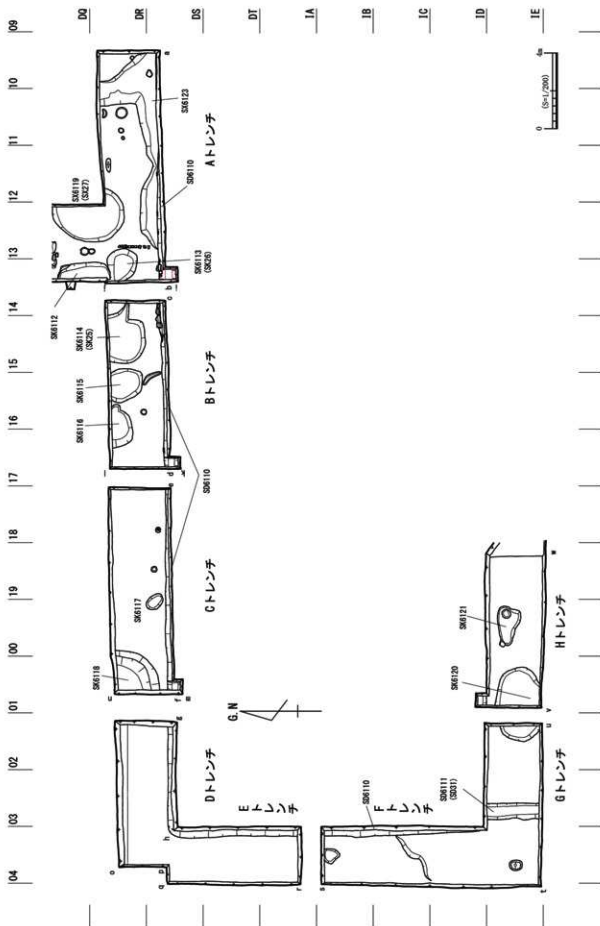
第8図 僧房跡覆屋排水地区 (S=1/200)
