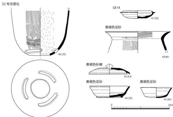
(1) 図3 32号住居跡・SX14・包含層出土遺物実測図(1:4)
