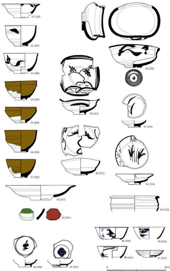
(3) 图2 SK1188出土遺物実測図(1:4)
