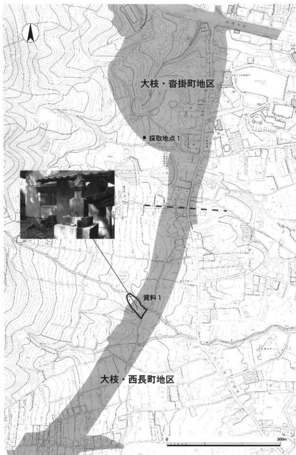
图6 採取地点1及び資料1位置図(1:5,000)
