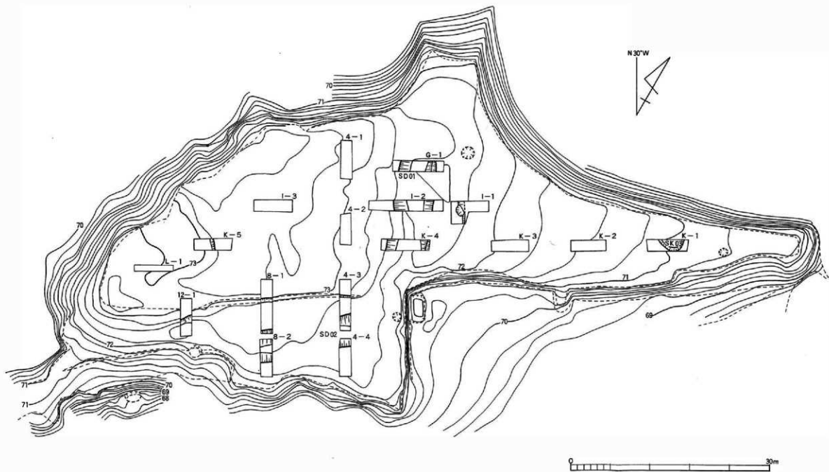
調查前地形圖 (試掘調査時)
