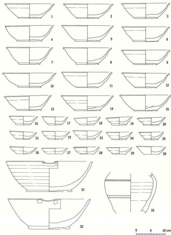
第27図 神明第2号竈窟内出土遺物実測図
