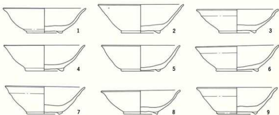
第38图 神明第1号窟分焰柱内出土遗物实测图
