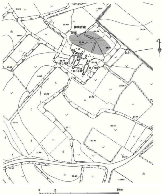
第16图 神明古窟発掘後地形図
