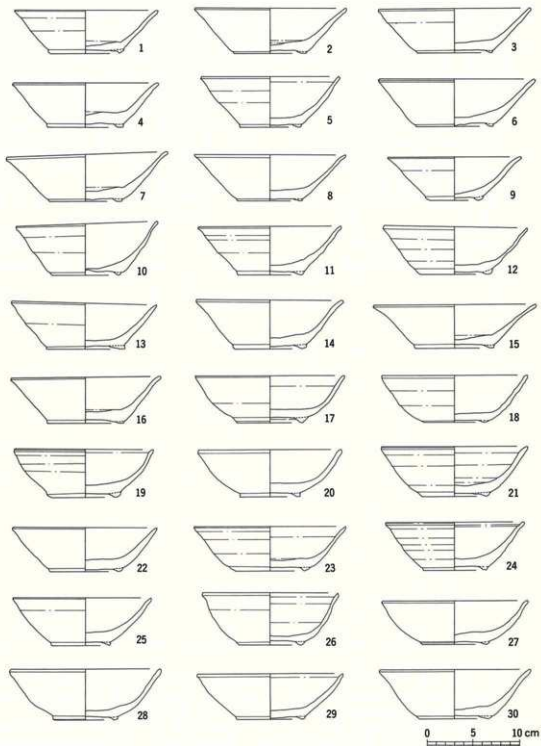
第13图 海陵庵古窟出土物实测图(1)
