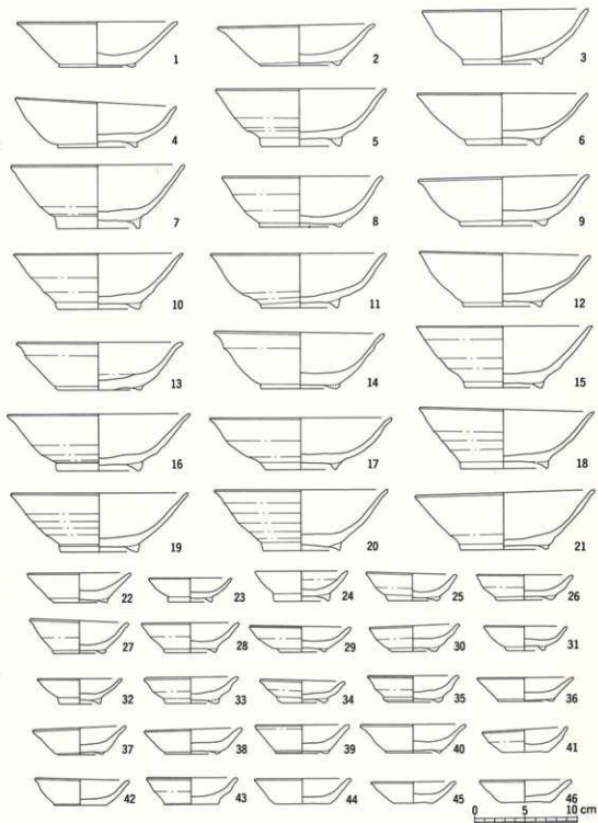
第36図 神明古窯灰原出土遺物実測図(1)
