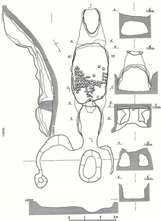
第18图 神明第2号窟窠体实测图
