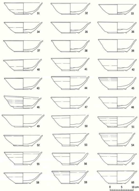
第14図 海陸庵古窯出土遺物実測図(2)
