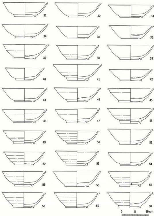
第33図 神明古窯前底部ベルト出土遺物実測図(2)
