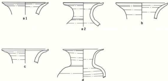
第26図 神明古窯出土の広口長頸瓶口縁端部器形分類図
