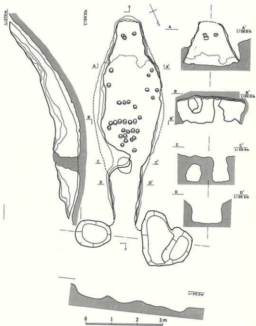
第19图 神明第3号窟窟体实测图
