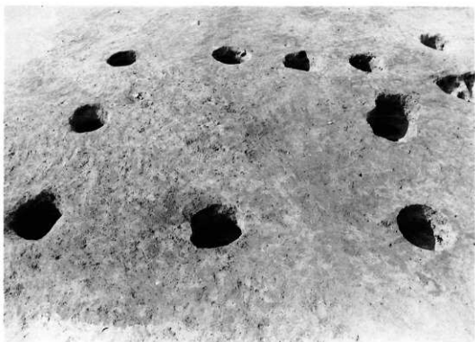
F-22号掘立柱建物址
