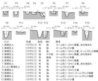
216号住居跡A・B柱穴想定図
