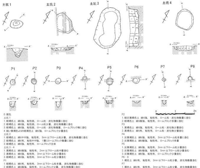
第72図 西ノ原遺跡第158地点土坑・ピット(1/60)
