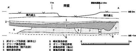
図45 遺構断面図 (1:40)
