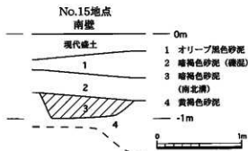
図33 Na15地点南北溝断面図 (1:40)
