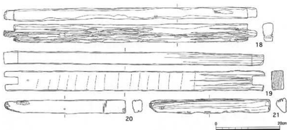
図11 井戸杵実測図(1:6)
