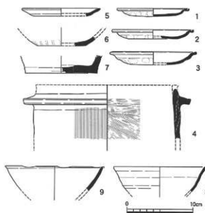
図4 出土遺物実測図 (1:4)
