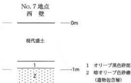
図30 No.7 地点柱状断面図 (1:40)
