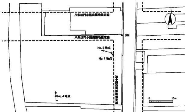
図7 遺構位置図 (1:500)
