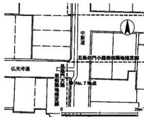
図29 遺構位置図 (1:500)
