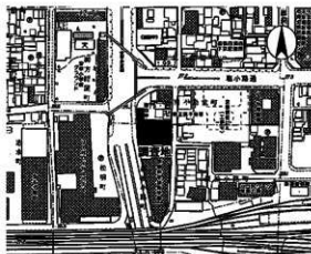
図6 調査位置図 (1:5,000)
