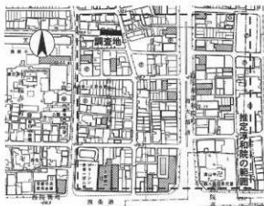
図16 調査位置図 (1:5,000)
