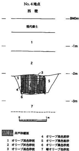
図9 No.4地点井戸断面図 (1:40)
