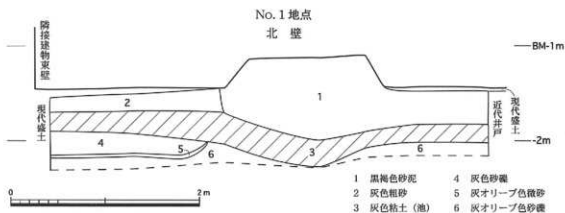
図3 No.1地点池断面図 (1:40)
