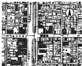
図1 調査位置図 (1:5,000)
