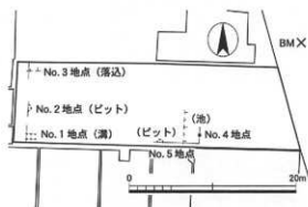
図17 遺構位置図 (1:500)
