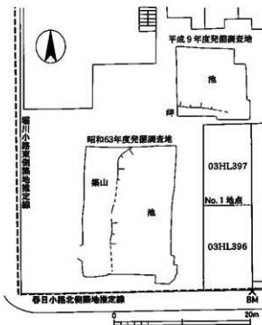
図2 遺構位置図 (1:500)
