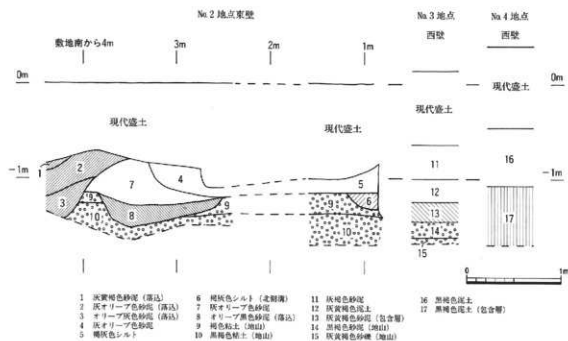
図12 遺構断面図 (1:4)
