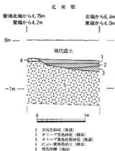
図23 遺構断面図 (1 : 40)
