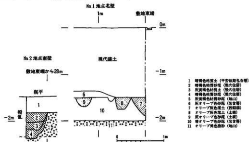
図17 遺構断面図 (1 : 40)
