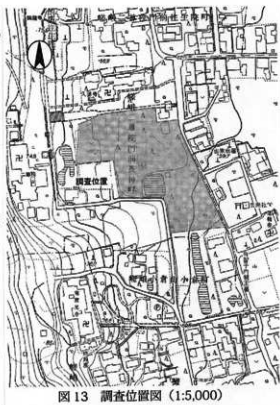
図13 調査位置図(1:5,000)
