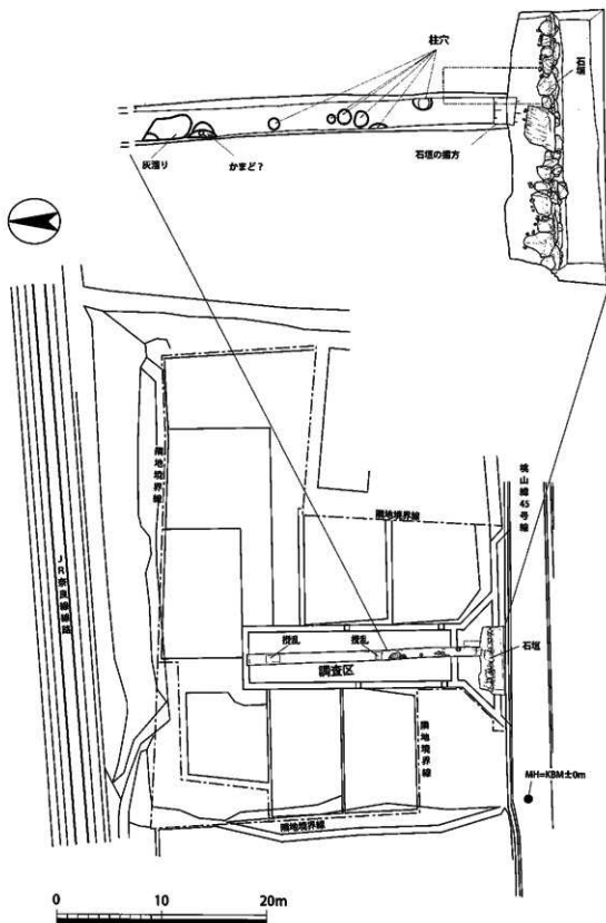
図26 試掘調査区位置図(1:400)・遺構検出図(1:100)
