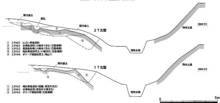
図21 各トレンチ土層断面図と残存土層断面図(1:100)
