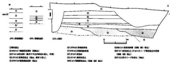
図 11 2・4トレンチ土層断面図 (1:50)
