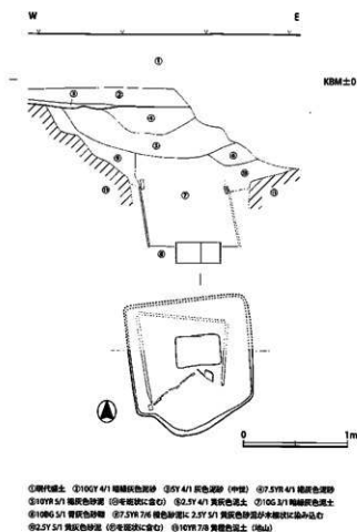
図 12 井戸 2 平・断面図 (1:40)
