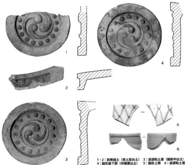
図 8 出土遺物写真及び実測図 (瓦のみ 1:3)
