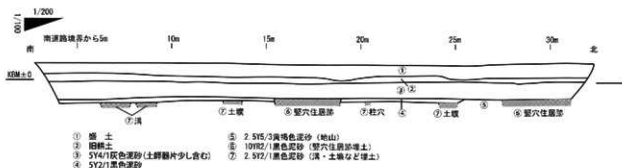
図24 トレンチ西壁土層断面図 (V=1:100 H=1:200)
