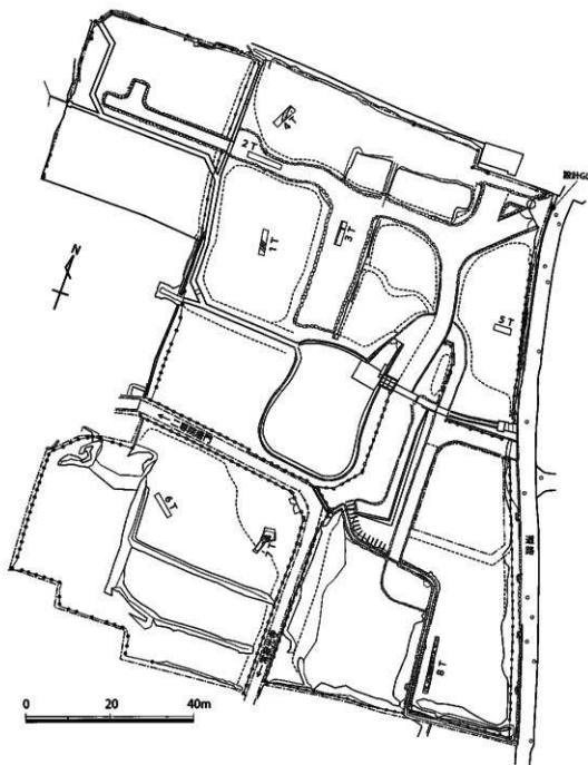
図 15 調査区位置図 (1:1,000)
