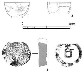
図28 出土陶磁器実測図（1:4）・泥面子実測図（1:1）
