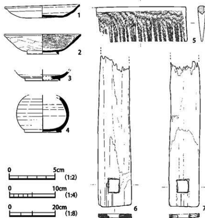
図13 出土遺物実測図（土器 1:4・櫛 1:2・部材 1:8）
