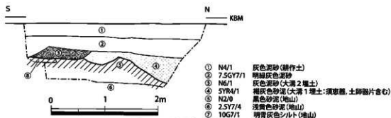
図34 5区西壁土層断面図 (1:50)
