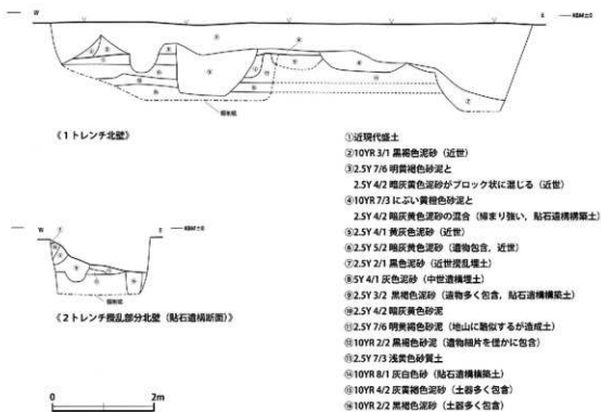
図5 土層断面図 (1:80)
