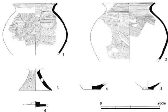
図36 出土遺物実測図 (S=1:4)
