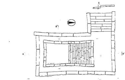
图7 水室平面及び断面実測図 (1:100)
