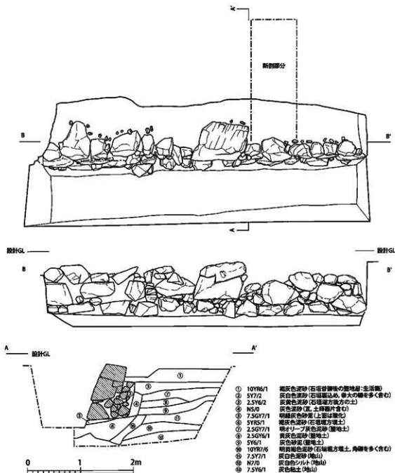
図 27 試掘調査拡張区平面図・立面図・断面図 (1:50)
