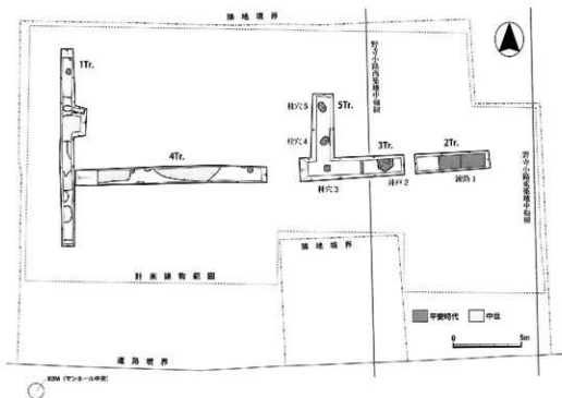
図10 調査区位置図 (1:300)
