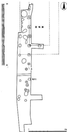
図12 遺構図 (1:250)
