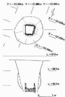
第28図 SE19 実測図
