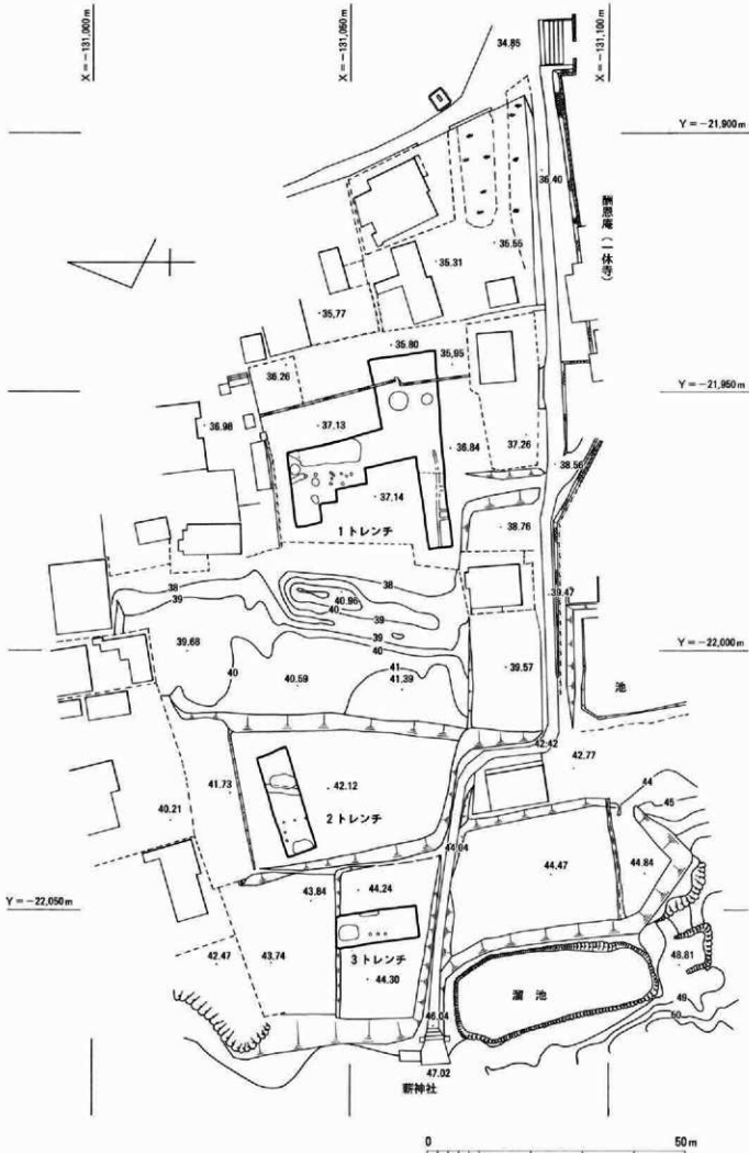
第8図 トレンチ配置図
