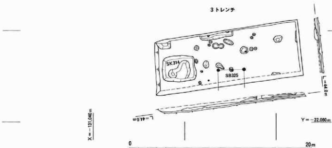
第34図 2・3トレンチ遺構図
