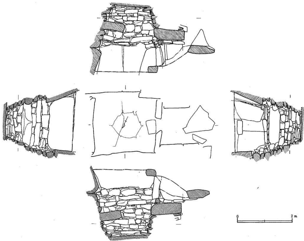
第3图 大松道古墳石室実測図
