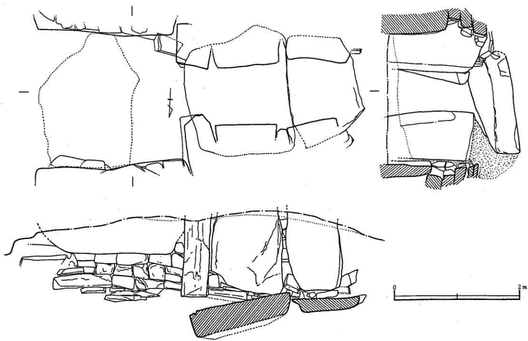
第4圖 金左衛門鬼塚古墳石室東測圖
