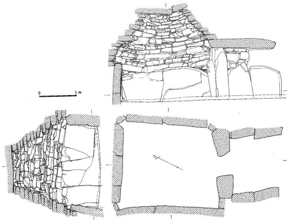
第16图 楠浦新田古墳石室夷面图
