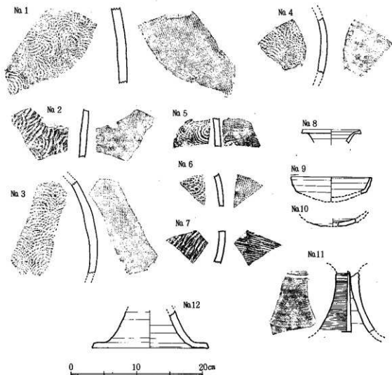
第14図 須森古墳表面採集遺物実測図
