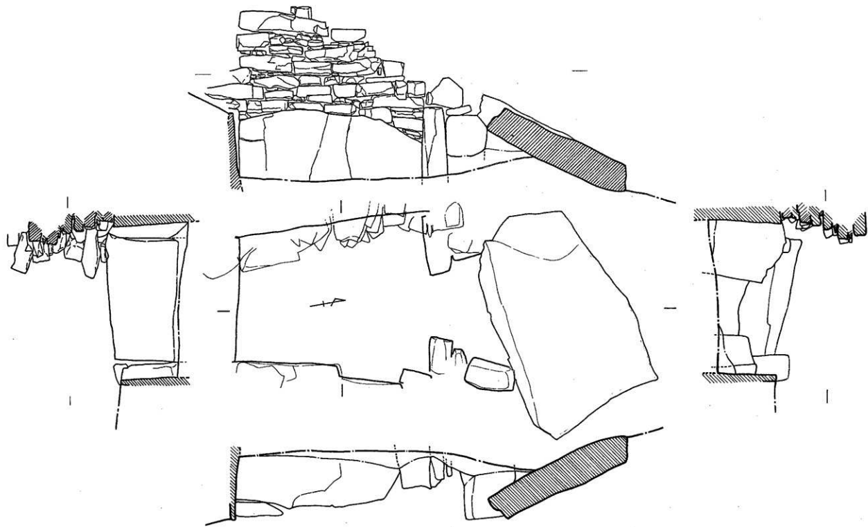
第5図 鬼の鼻古墳石室実測図
