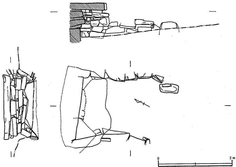
第7图 观音向山1号填石室实测图
