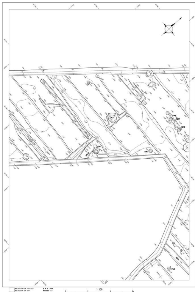
第 186 図 直江北遺跡 遺構平面図 No.68 (S=1/100)
