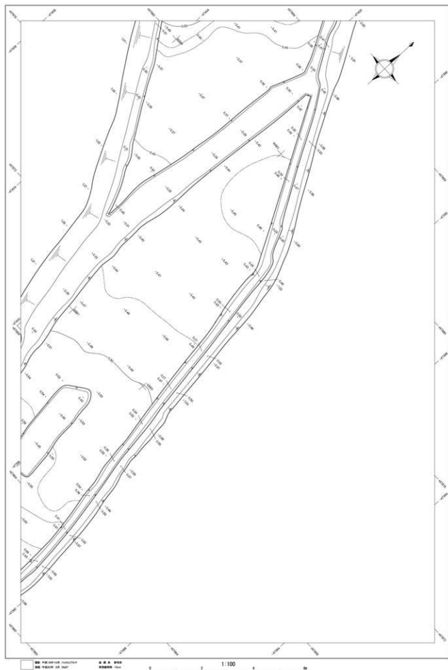
第 205 図 直江北遺跡 遺構平面図 No.87 (S=1/100)
