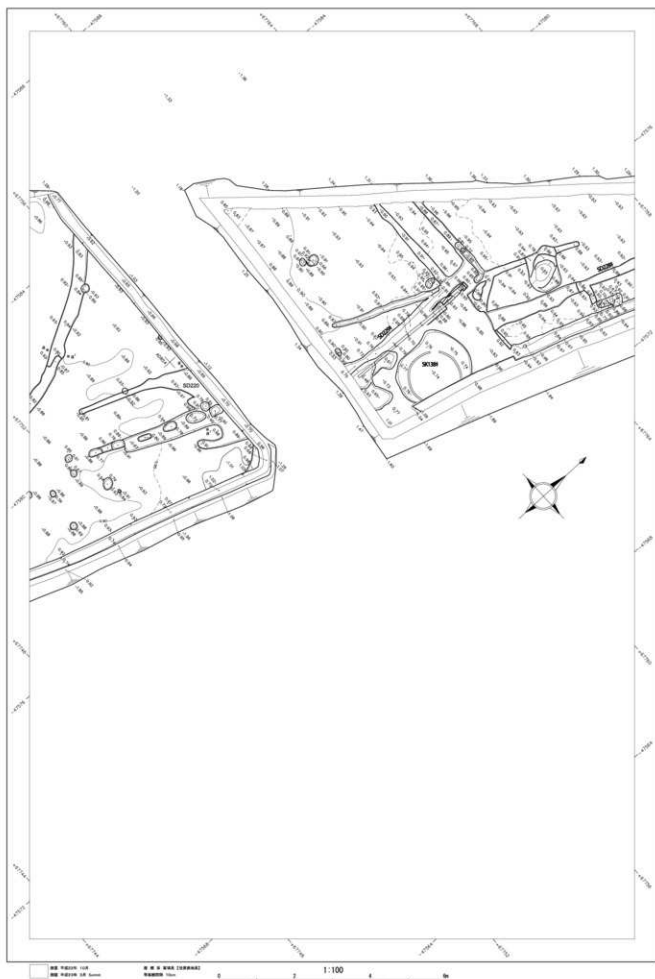
第177図 直江北遺跡 遺構平面図 No.59 (S=1/100)
