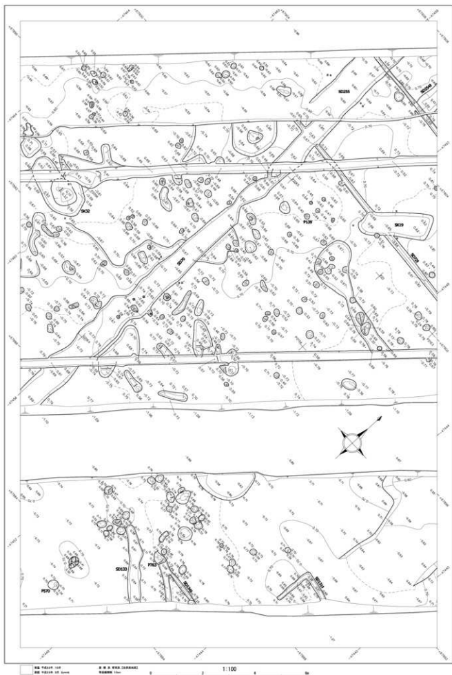
第 170 図 直江北遺跡 遺構平面図 No.52 (S=1/100)
