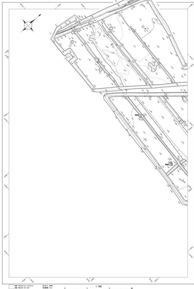
第 182 図 直江北遺跡 遺構平面図 No.64 (S=1/100)
