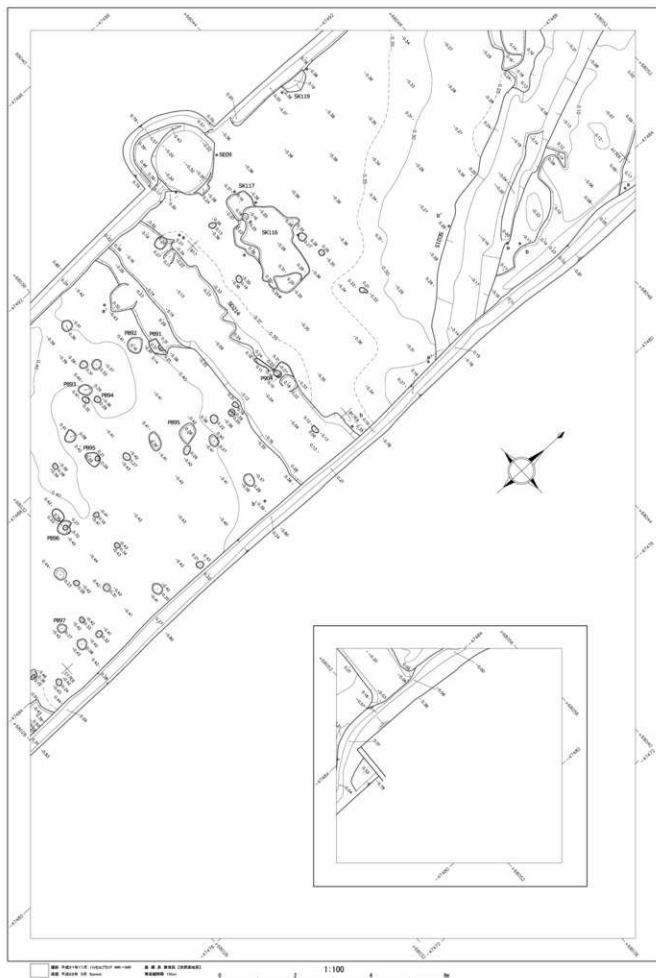
第 122 図 直江北遺跡 遺構平面図 No.4 (S=1/100)
