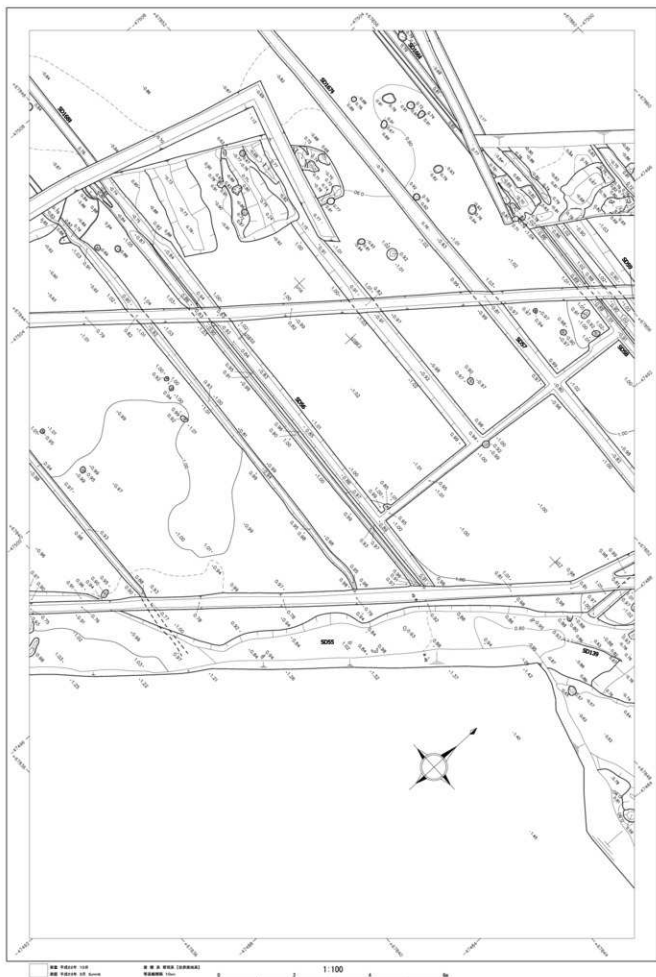
第 166 圖 直江北遺跡 遺構平面圖 No.48 (S=1/100)
