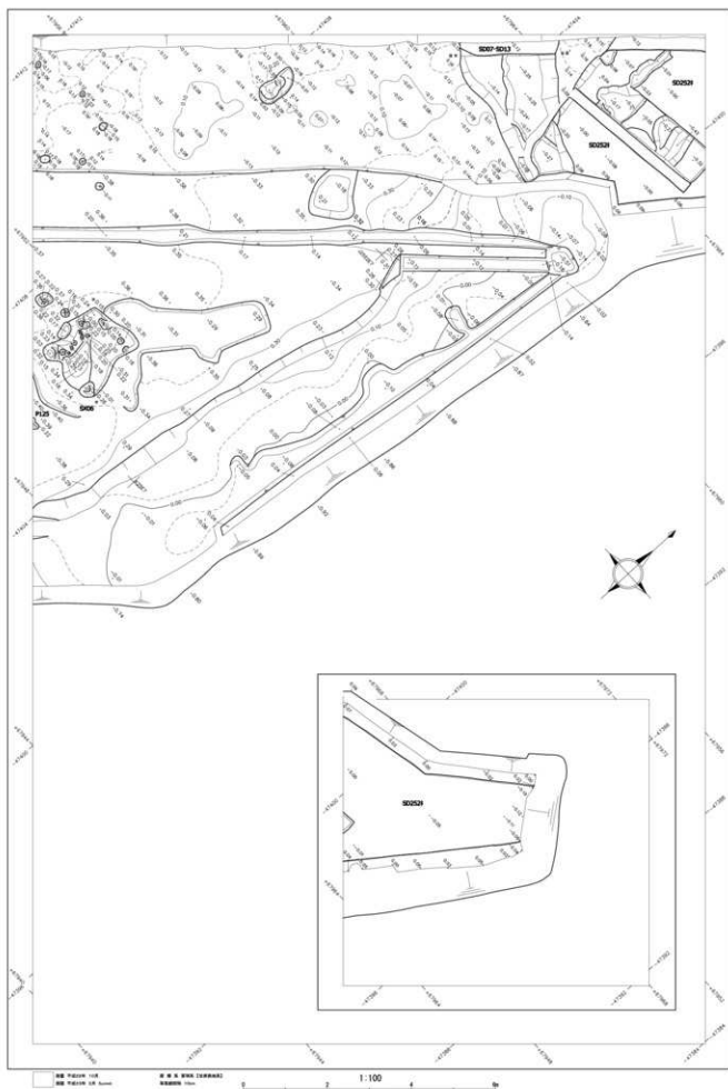
第175図 直江北遺跡 遺構平面図 No.57 (S=1/100)
