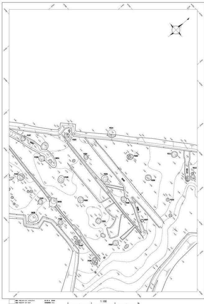
第 196 図 直江北遺跡 遺構平面図 No.78 (S=1/100)
