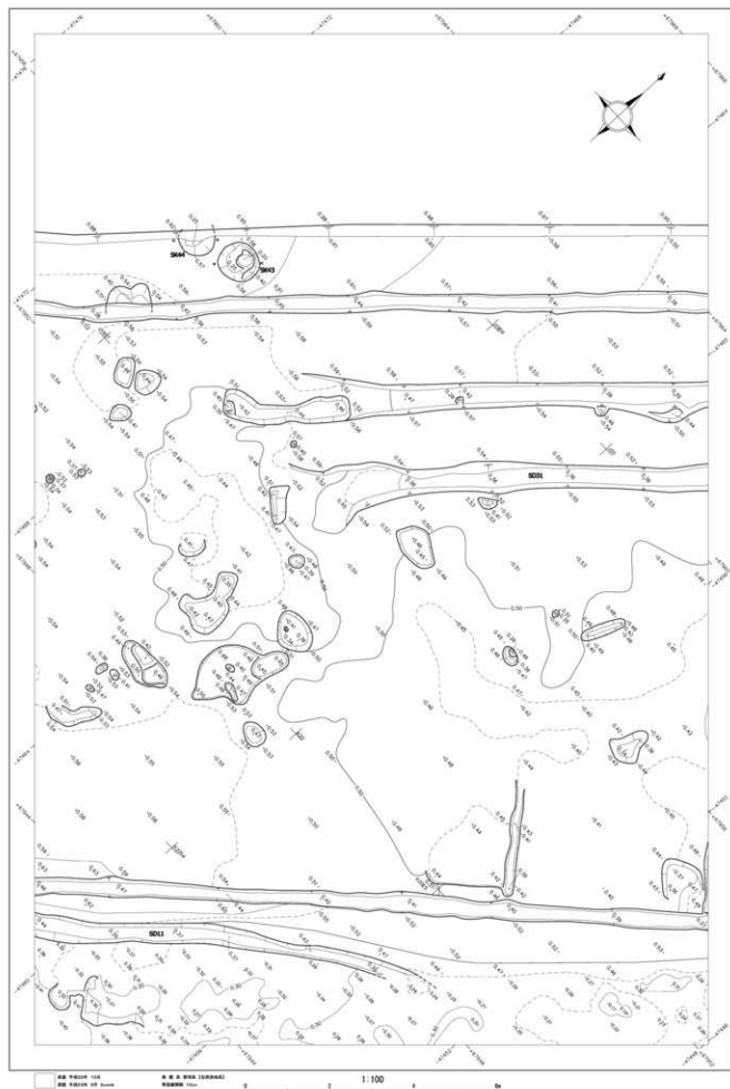
第145 図 直江北遺跡 遺構平面図 No.27 (S=1/100)
