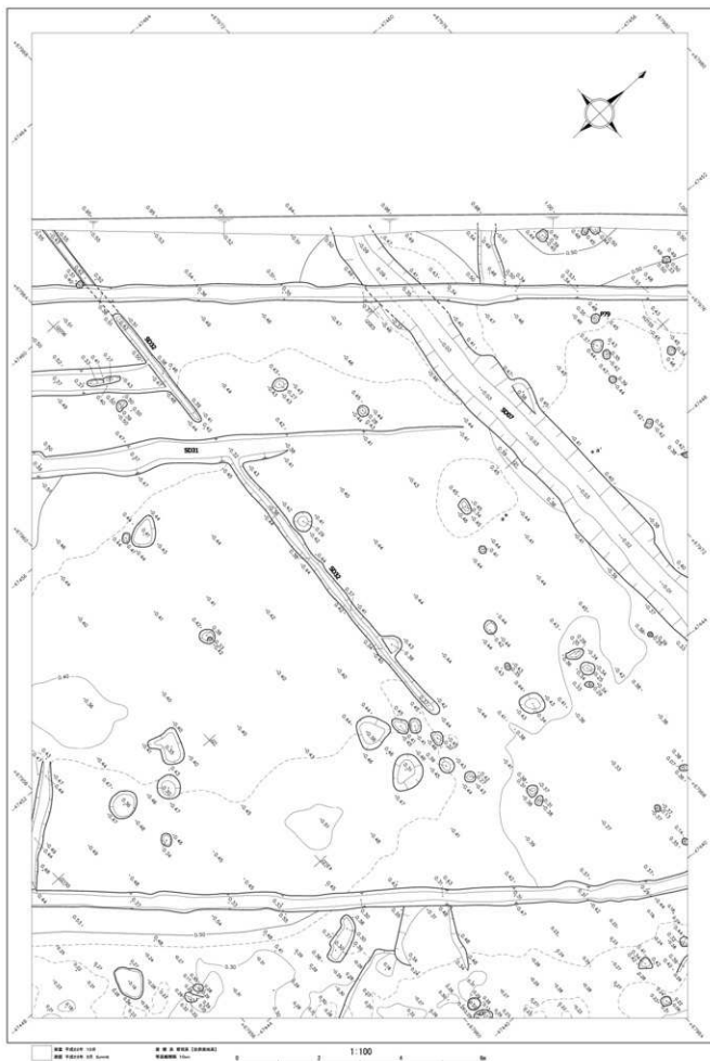
第 146 図 直江北遺跡 遺構平面図 No.28 (S=1/100)
