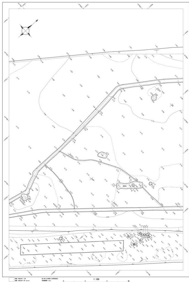
第133図 直江北遺跡 遺構平面図 No.15 (S=1/100)
