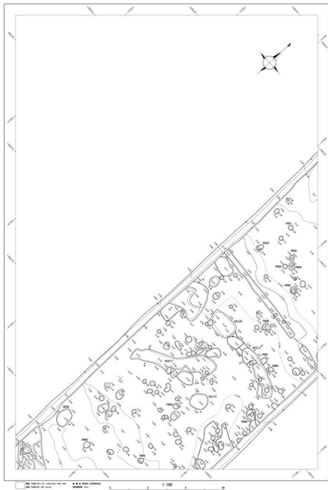
第121図 直江北遺跡 遺構平面図 No.3 (S=1/100)
