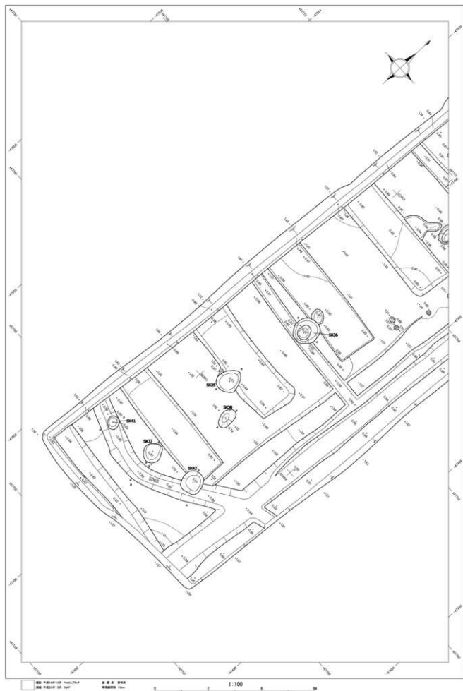
第199 図 直江北遺跡 遺構平面図 No.81 (S=1/100)
