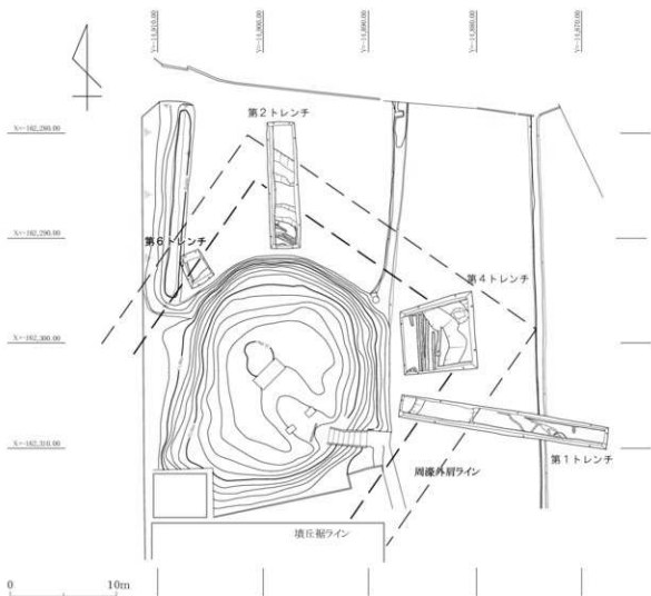
図20 墳丘復元図 (S=1/400)
