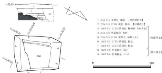
図16 第6トレンチ平面・断面図 (S=1/80)
