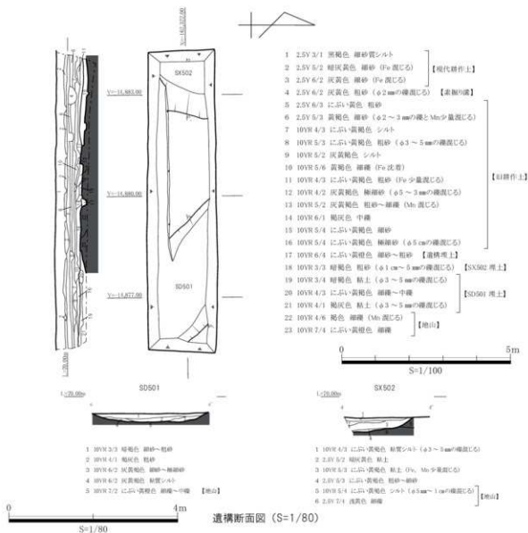
図15 第5トレンチ平面・断面図 (S=1/100)
