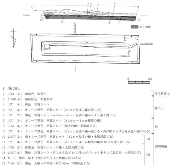
図4 調査区平面・断面図 (S=1/150)
