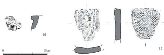
図6 出土瓦 (S=1/4)
