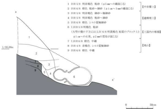
図22 調査区平面・断面図 (S=1/20)
