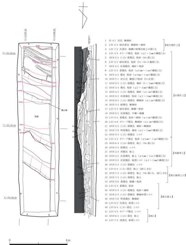
図12 第2トレンチ平面・断面図 (S=1/80)
