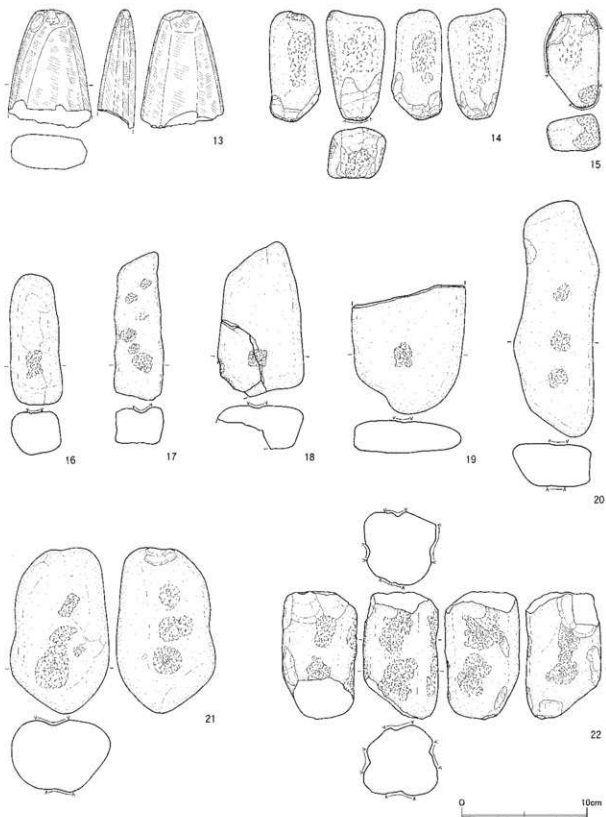
図Ⅲ-8 包含層（V層）出土の石器（2）
