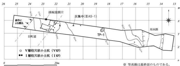
図 I-3 遺構位置図
