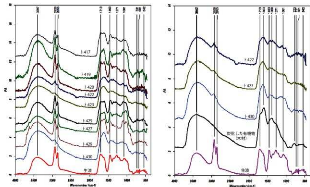
漆状物質のIRスペクトル
