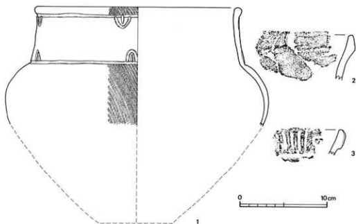
Fig 16 縄文土器実測図 (1 : 3)
