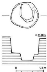
Fig 13 P 11 実測図 (1 : 20)
