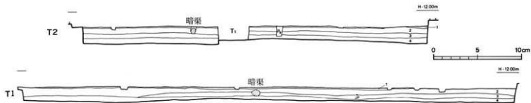
Fig 6 T1, T2セクション図 (1:120)
