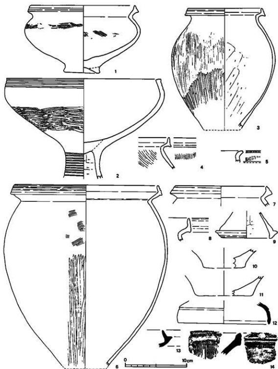
Fig 18 弥生土器，須惠器実画図（1：3）
