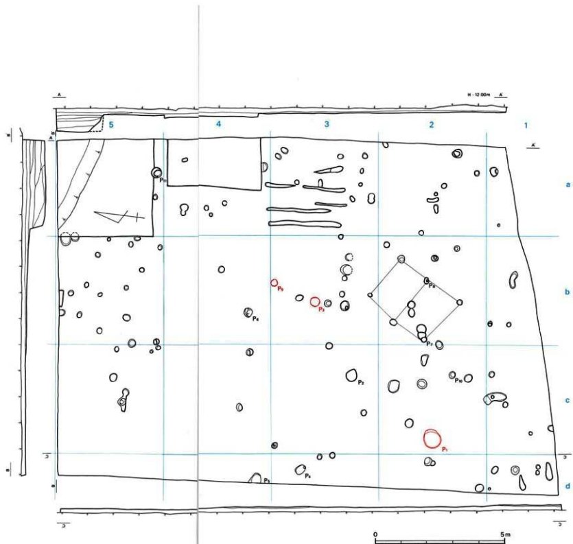
Fig 11 遺構配置図 (1 : 100, 青は弥生時代中期, ピット番号は記述上必要なもののみ付した)
