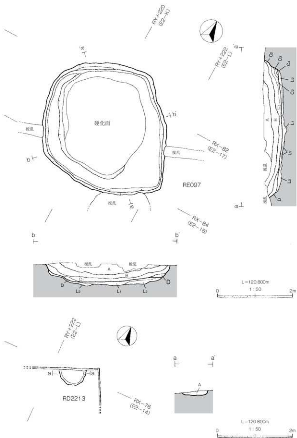
第 14 図 RE 097 竪穴跡・RD 2213 土坑
