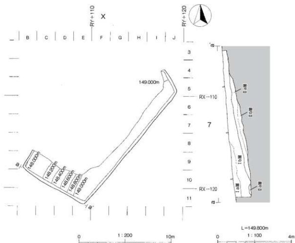
第18図 西黒石野遺跡第14次調査全体図
