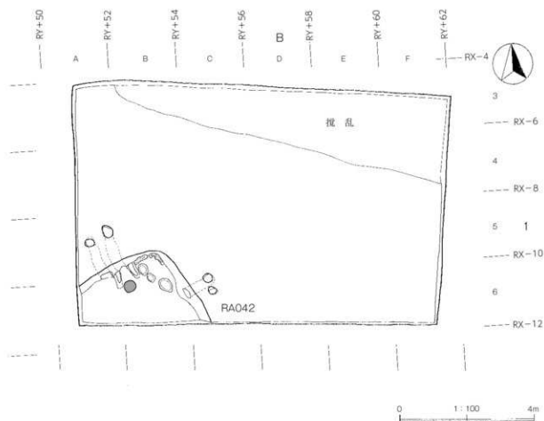
第 4 図 西鹿渡遺跡第 30 次調査全体図
