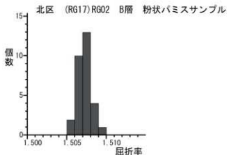
図1 火山ガラスの屈折率
