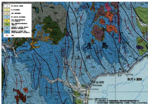
図Ⅱ-2 木古内町周辺の地質
