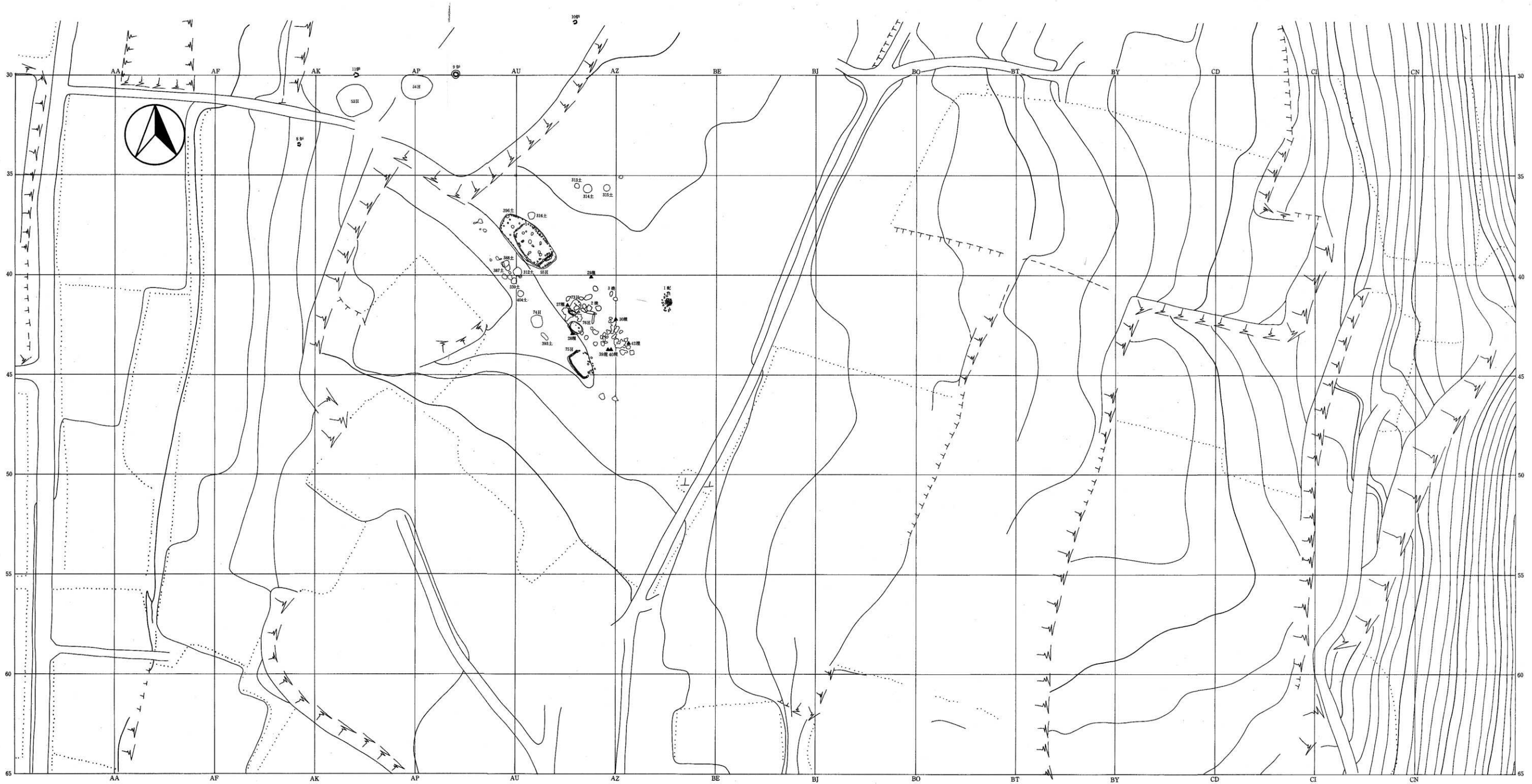
付図2 畑内遺跡遺構配置図② (S=1/400)
