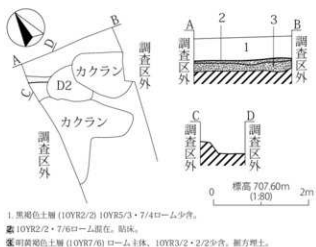
第13図 H11号住居址
