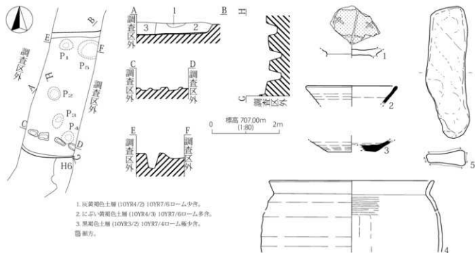
第11図 H9号住居址
