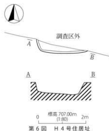
第6図 H4号住居址
