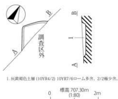
第12図 H10号住居址
