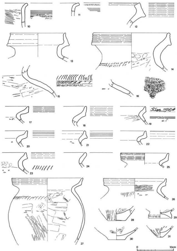
第9图 调查区内出土物实测图I (1:3) 弥生土器
