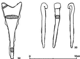
第10図 調査区内出土遺物実測図Ⅱ(1:2) 鉄器
