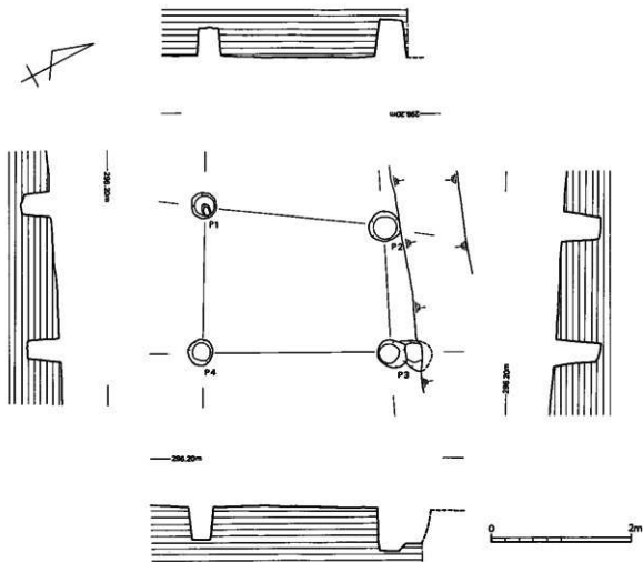
第7図 SB 3 実測図 (1:60)
