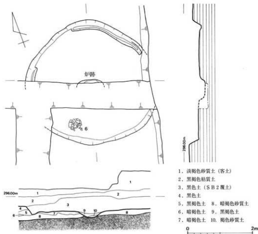
第5図 SB 2実測図(1:60)
