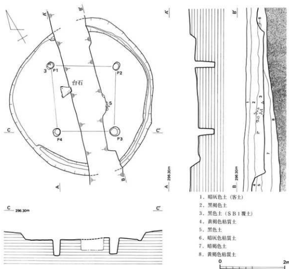
第4図 SB1実測図(1:60)
