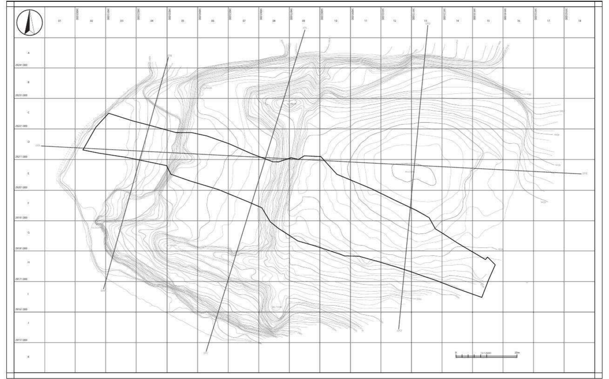
地形測量図
