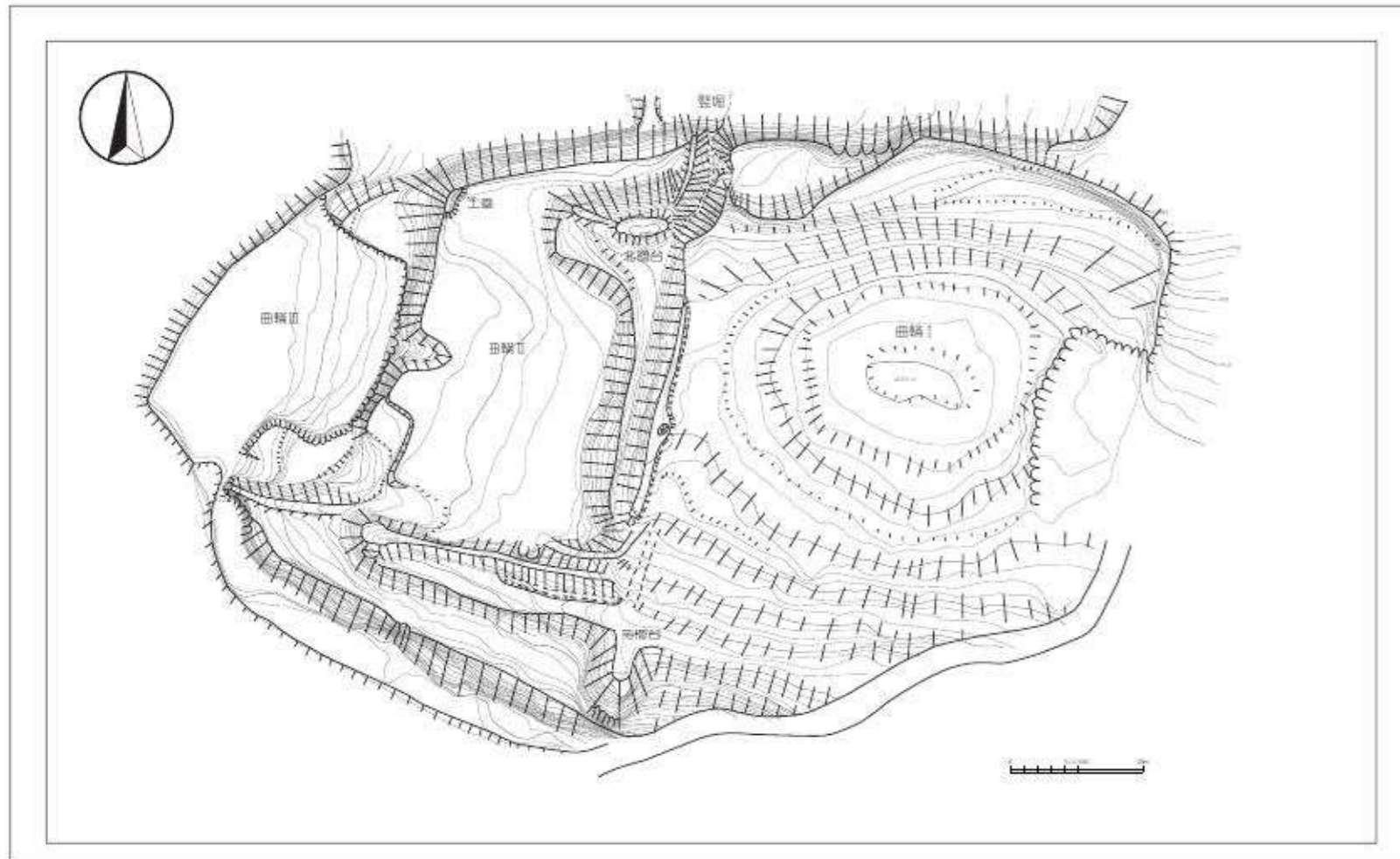
縄張図
