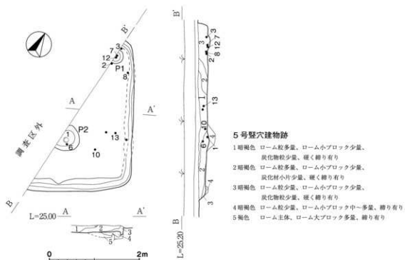
第8図 5号竪穴建物跡
