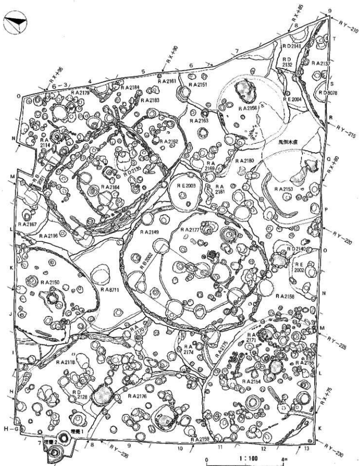
大船町遺跡 第37次調査区全体図 (1:100)
