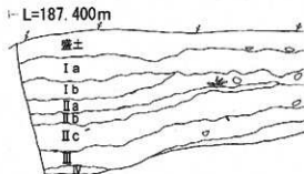
第3図 第36次調査区南西隅土層図 1:60
