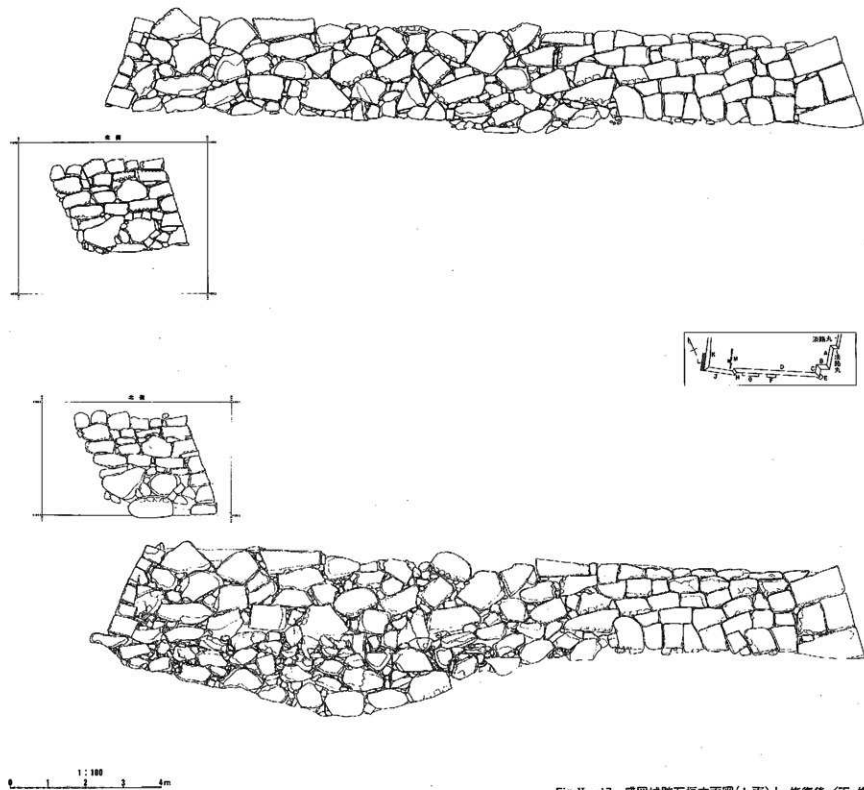
Fig. V-17 盛岡城跡石垣立面図(L面)上・修復後/下・修復前
