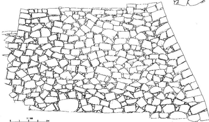
Fig. V - 16 盛岡城跡石垣立面図(K面)上・修復後/下・修復前
