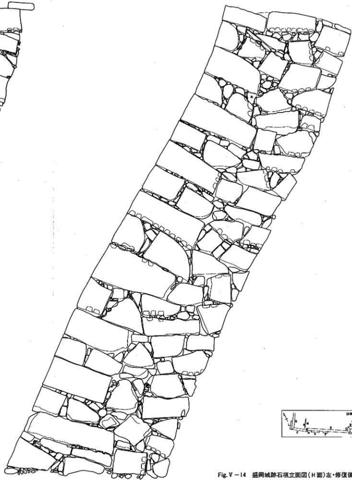
Fig. V-14 盛岡城跡石垣立面圖(H面)左・修復後/右・修復前
