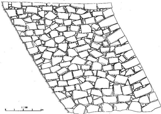
Fig. V-11 盛岡城跡石垣立面図(B面)上・修復後/下・修復前
