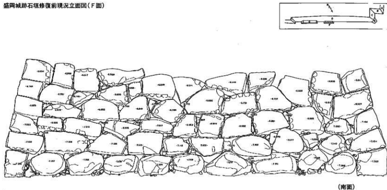
盛岡城跡石垣修復前現況立面圖 (F面)
