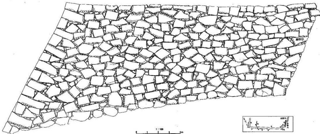
Fig. V-10 盛岡城跡石垣立面図(A面)上・修復後/下・修復前
