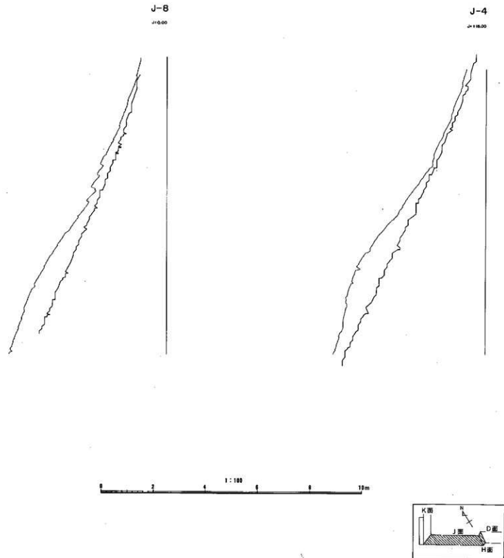
Fig.V - 22 盛岡城跡石垣構断面(H、J面)修復前(細線)・後(太線)
