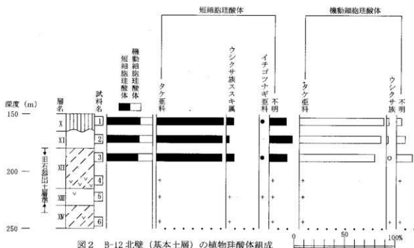
図2 B-12北壁（基本土層）の植物珪酸体組成
