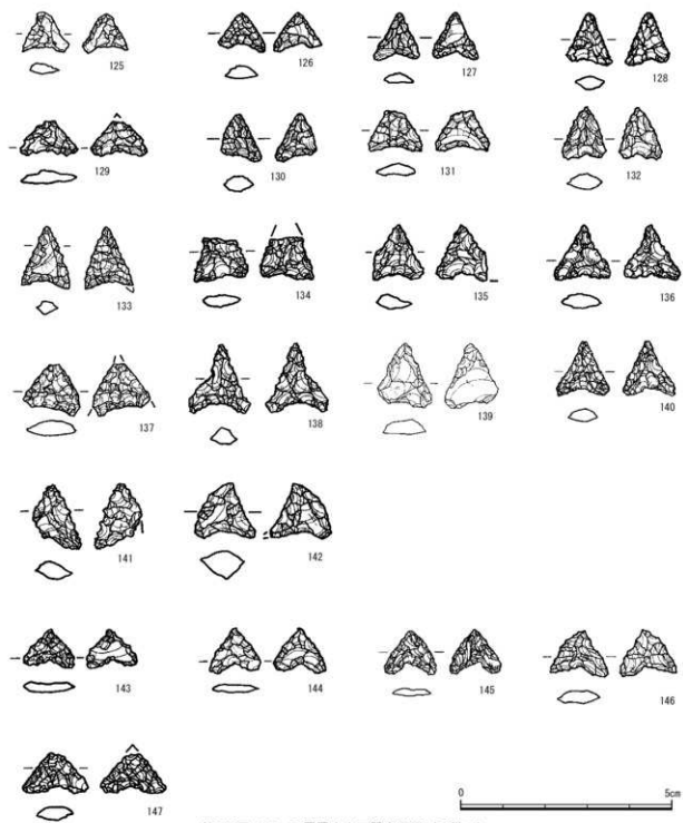
第399圖 VI~VII層層出土石器実測図（石鏃3）
