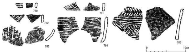
第384図 X II類土器実測図
