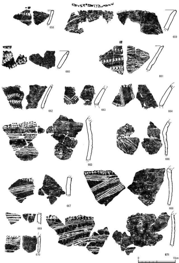
第366圖 X類土器実測圖(16)
