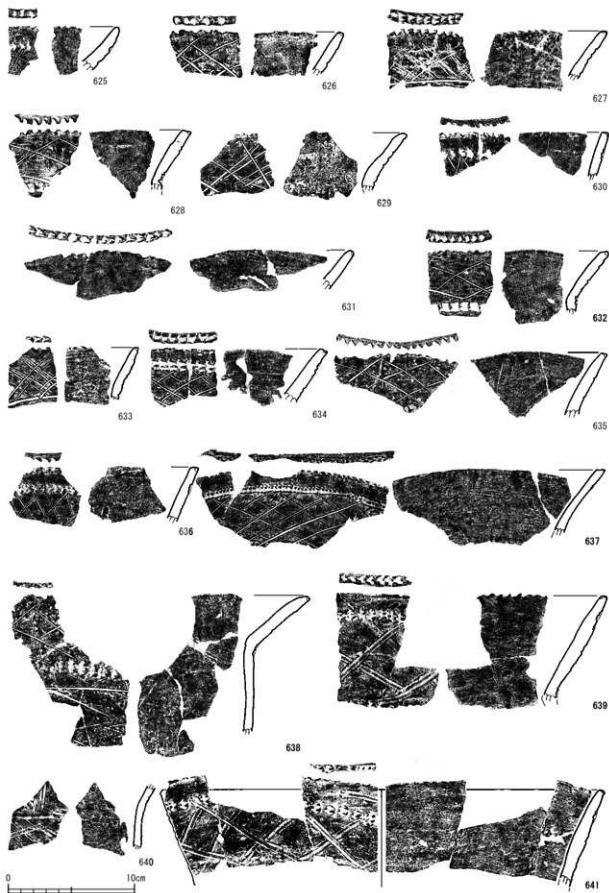
第362图 X類土器実測図(12)
