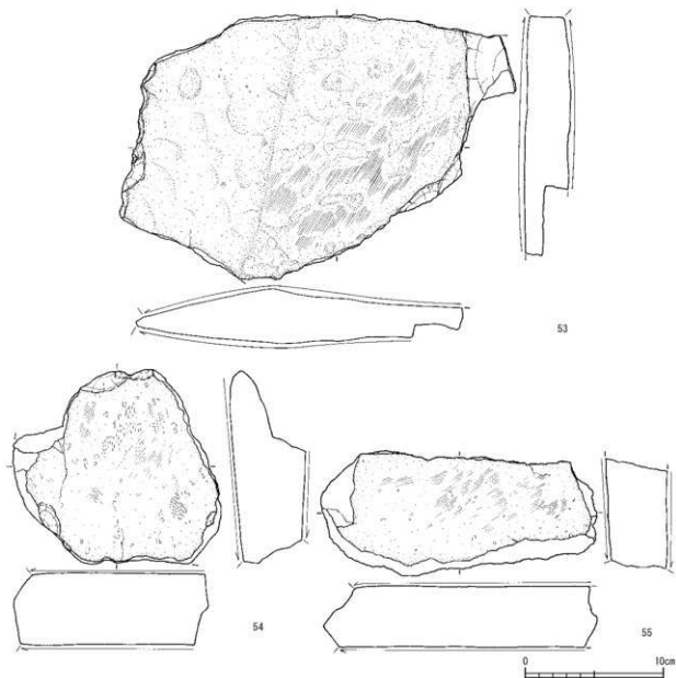
第394図 Ⅷ層出土石器実測図（石皿）
