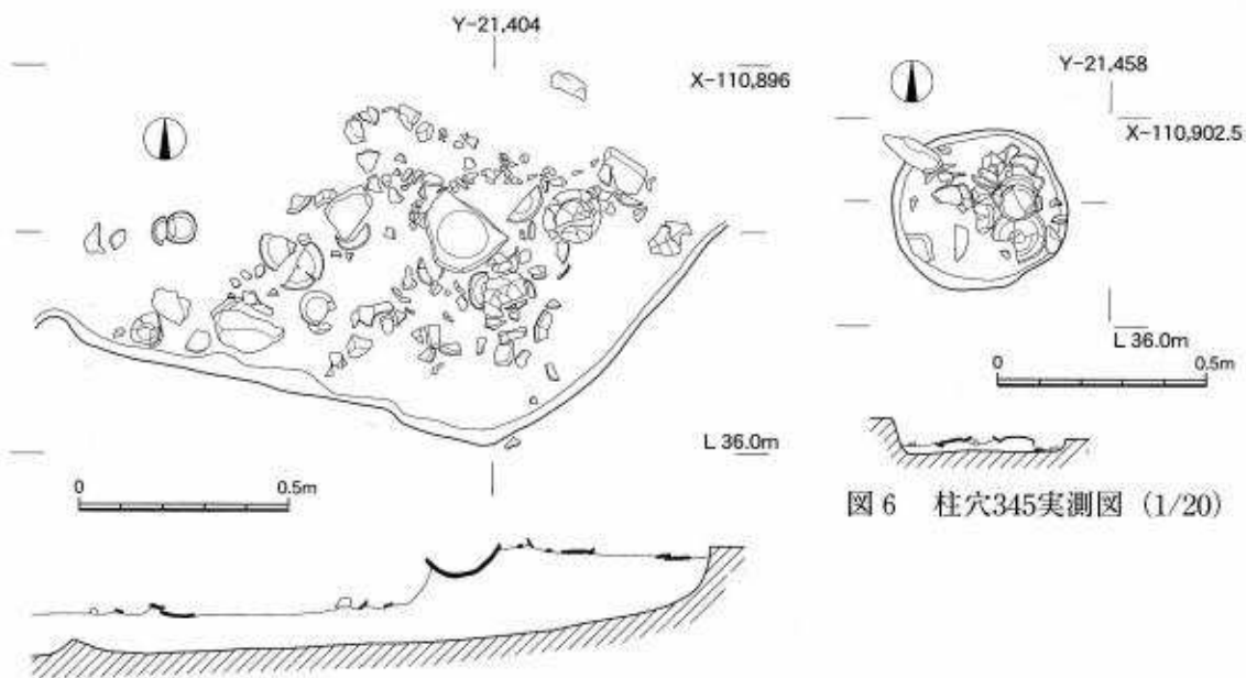
図5 土塋163実測図 (1/20)
