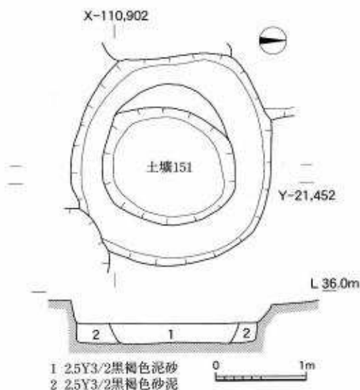
図12 土壙151実測図 (1/60)
