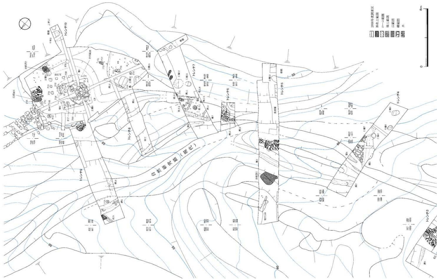
第4図 トレンチ4～10・荒神堂跡 遺構配置図
