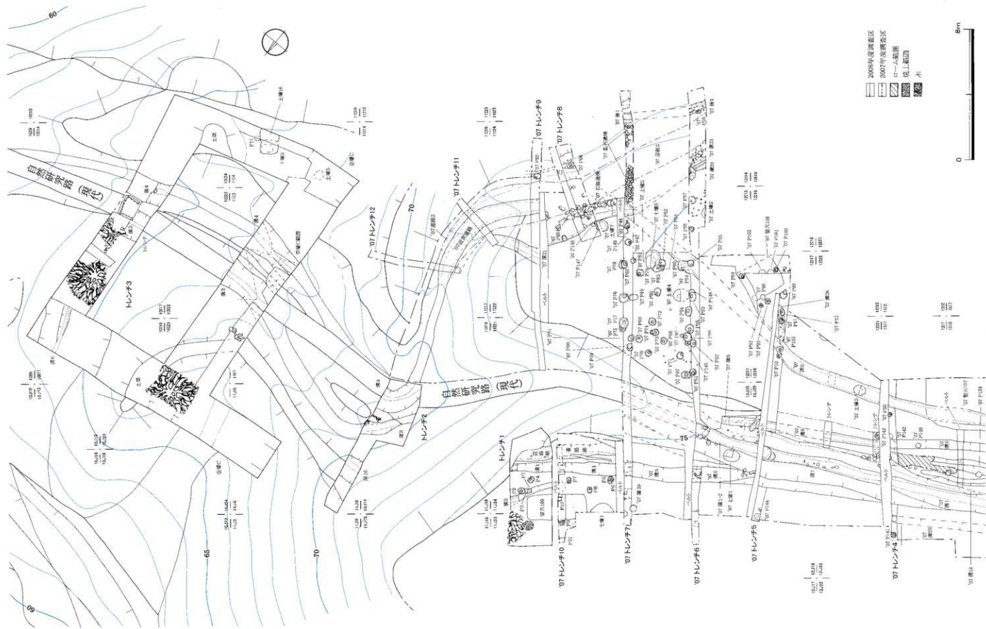
第3図 '07年度調査区・トレンチ1～3 遺構配置図
