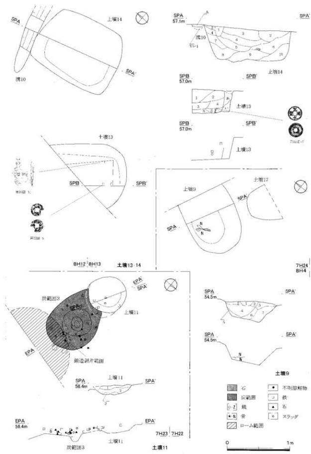
第15図 土壇 9・11・13・14・17 溝10 炭範囲3 遺構平面図他
