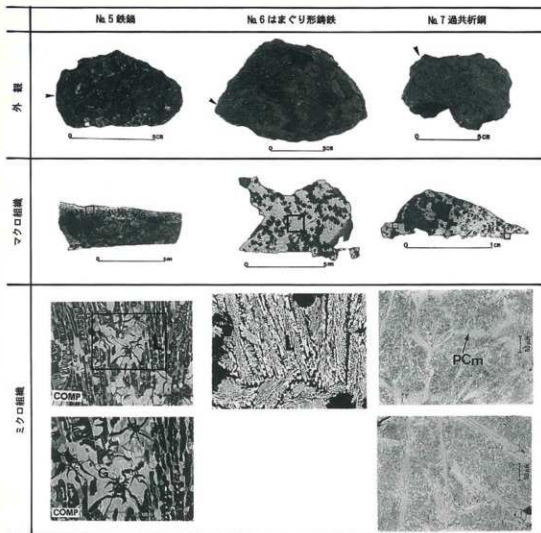
図3 No. 5 鉄鍋・No. 6 はまぐり形鋳鉄・No. 7 過共析鋼の外観と抽出した試料片の組織観察結果 外観の矢印は試料片抽出位置。No. 6・No. 7 はナイトールによるエッチングを実施。 マクロまたはマクロエッチング組織の枠囲んだ内部をミクロ組織観察。COMPはEPMAによる組成像。 Lはレーアブライト組織、Gは片状黒鉛、PCmは初析セメントライト。
