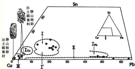
図9 輸入明銭と国内横鑄銭の化学成分組成範囲の概念図
