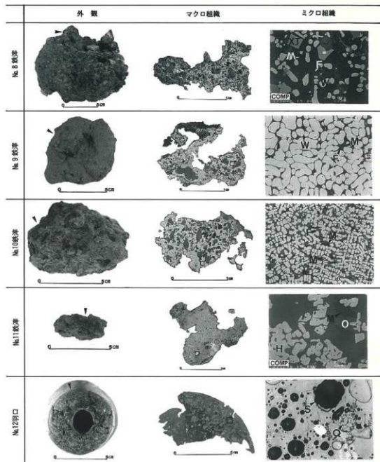
図4 鉄滓・羽口の外観と抽出した試料片の組織観察結果
