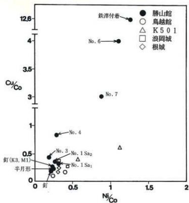
図8 出土鉄器・鉄塊のCu, Ni, Co成分比
