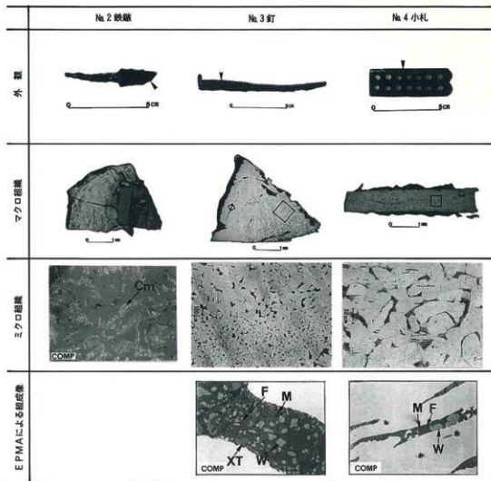
図2 鉄器の外観と抽出した試料片の組織観察結果
