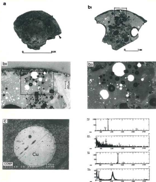
図5 No.15るつぼの外観と抽出した試料片の組織観察結果
