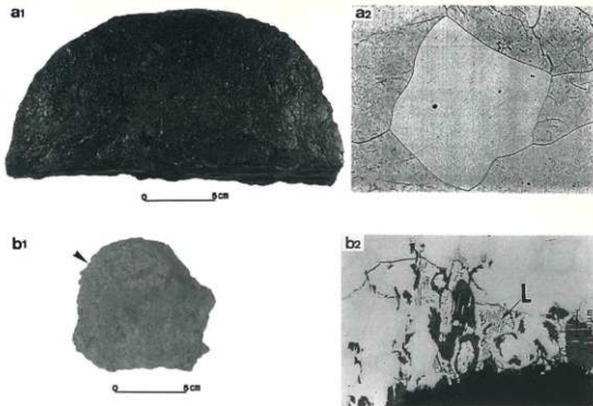
図6 半月形鉄塊ならびに鉄塊系遺物の外観と組織観察結果
