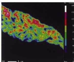
写真1 No.1 (7026) 半製品の非金属介在物に含有される元素濃度分布のカラーマップ 色が青-赤-白の順に含有濃度が高い。 XTは鉄チタン酸化物、FはFeO-MgO-SiO 2 系化合物、Mはマトリクス。
