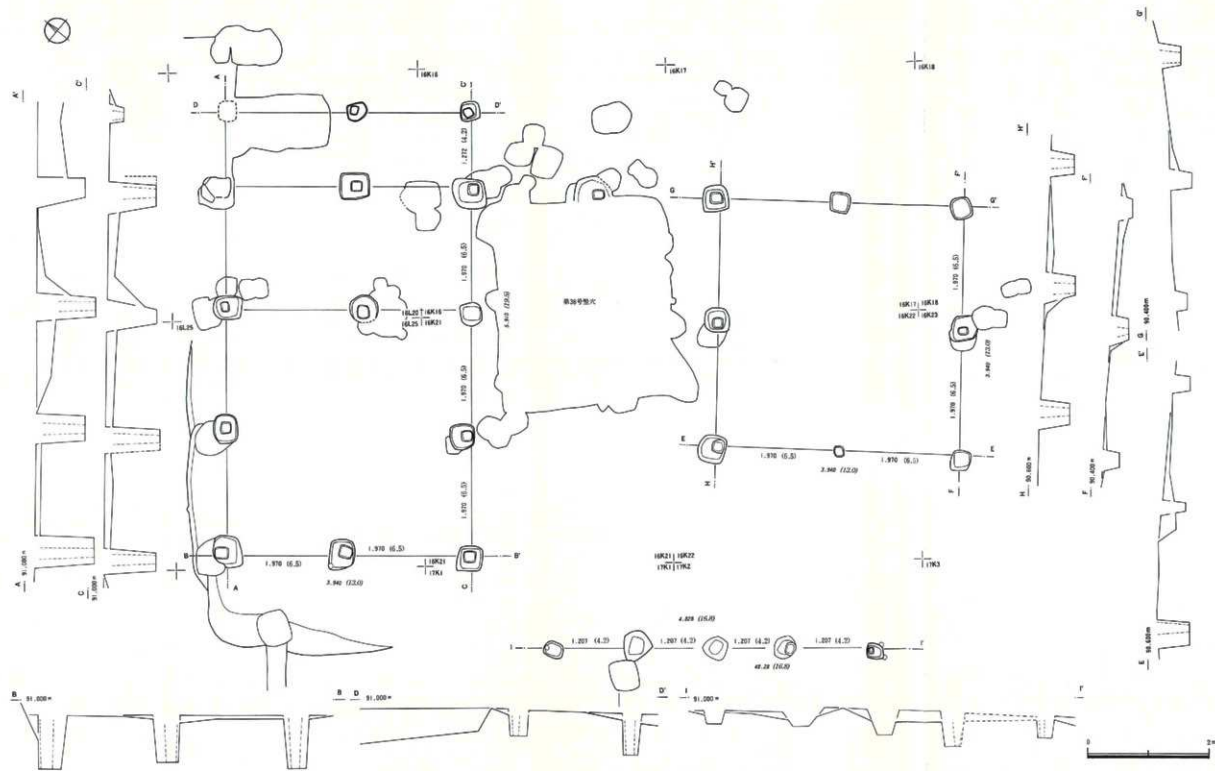
第19图 第3号·第4号建筑物想定图
