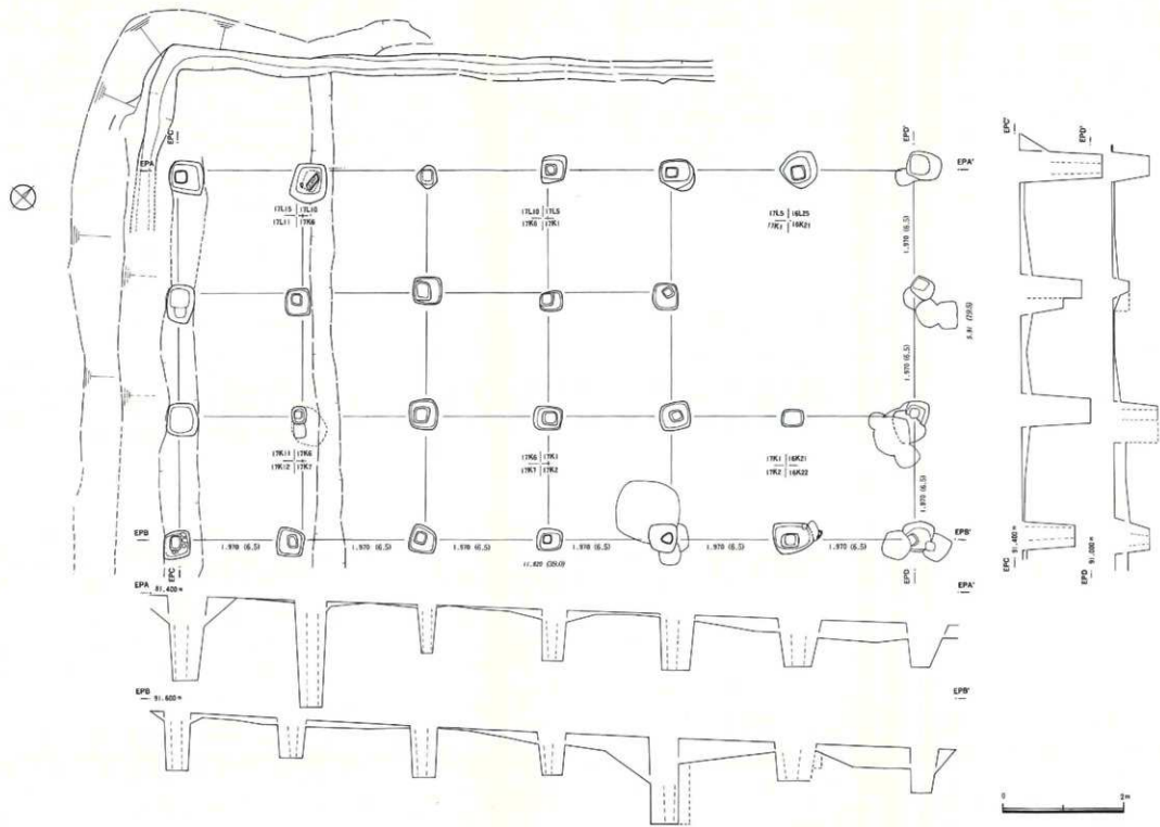
第20图 第5号建物跡想定図
