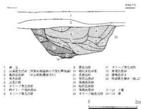
図13 1トレンチ西壁土塼断面図（1：80）
