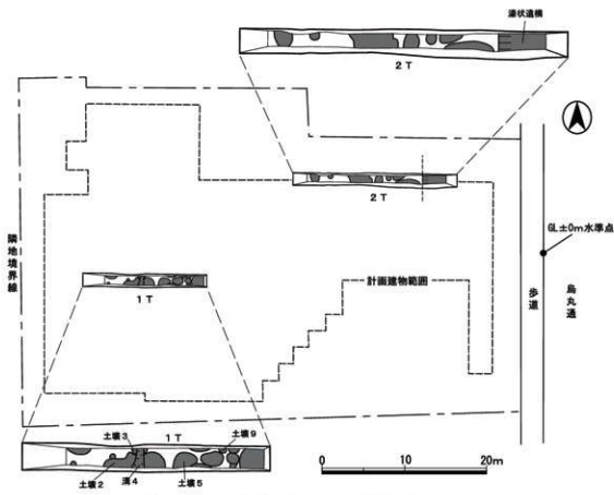
図16 トレンチ位置図 (1:500)・遺構平面図 (1:250)
