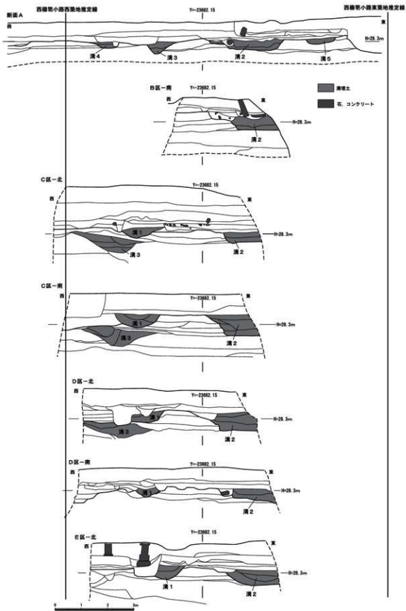
図26 土層比較図 (1:100)
