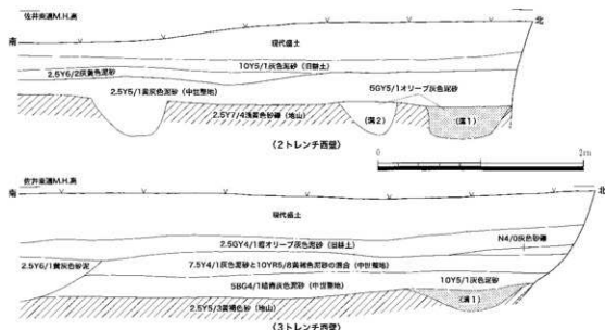
図35 土層断面図 (1:40)
