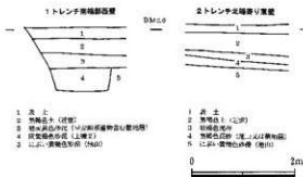
図4 各トレンチ土層図 (180)
