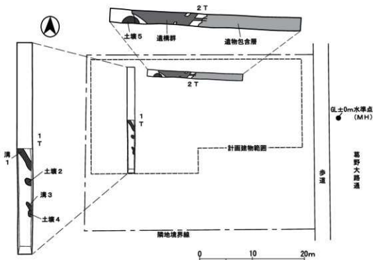
図29 トレンチ位置図(1:500)・遺構平面図(1:250)
