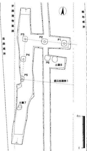
図40 遺構平面図 (1:130)
