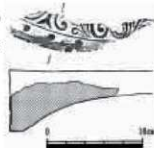
図45 出土軒平瓦 (1:4)
