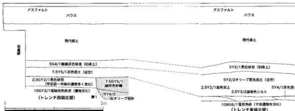
図22 土層断面図 (1:40)
