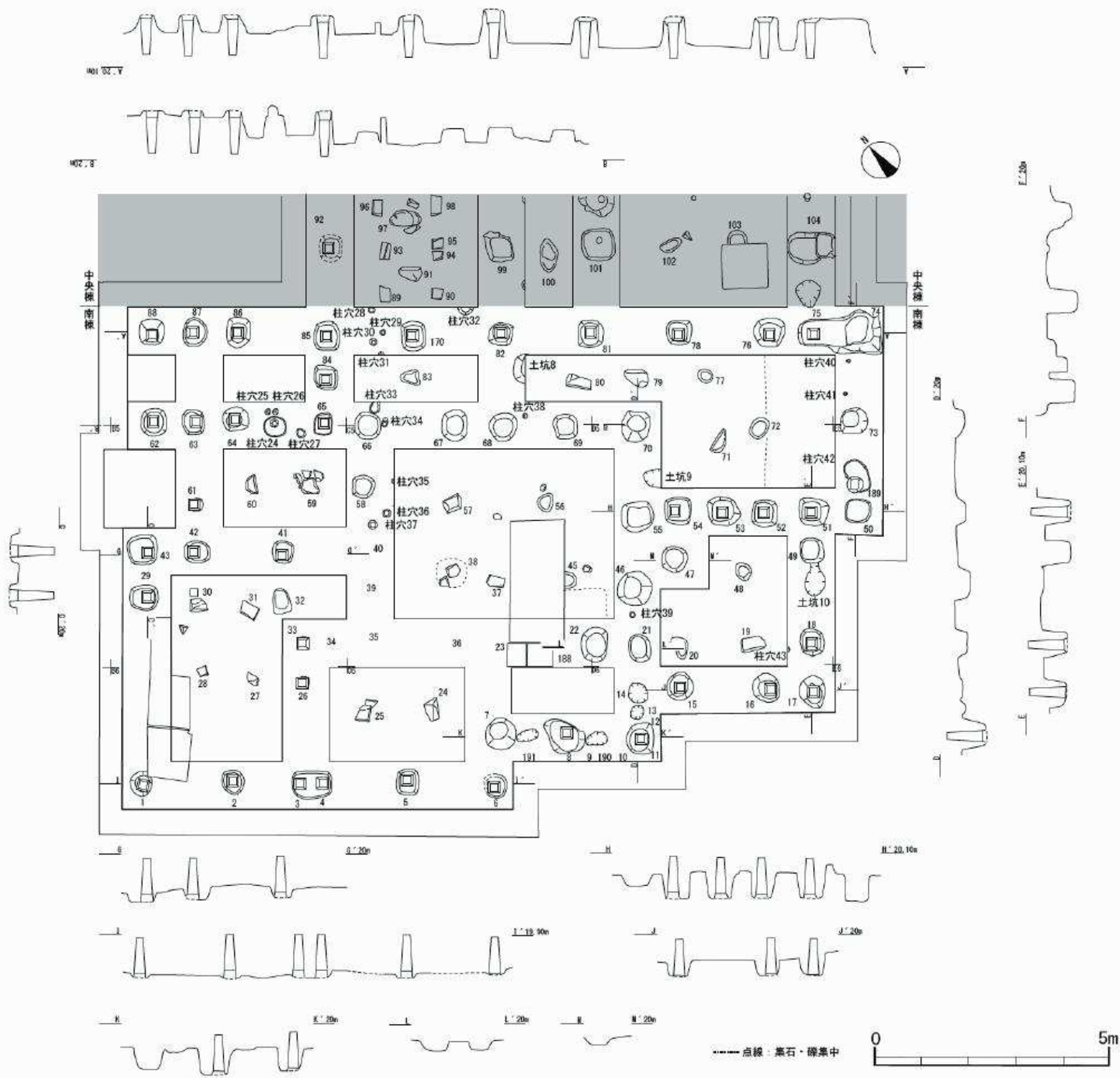
第19图 南棟実測図
