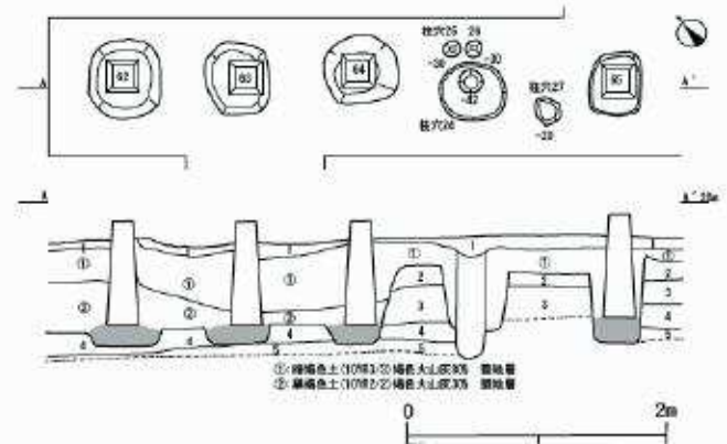
第21図 南棟礎石地業検出状況 (礎石番号:62・63・64・65)
