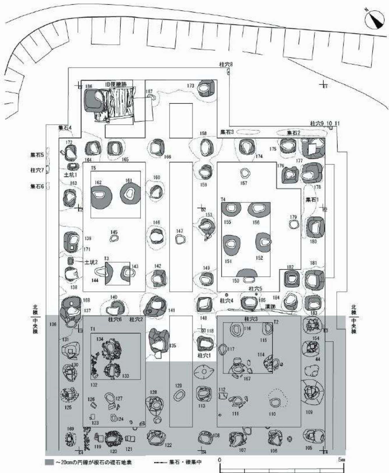
第8図 北棟造構配置図
