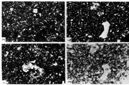
Plate 2 N-2. 須惠器 (環) 出土地: 江釣子村猫谷地 1: 文象斑岩。(偏光ニコル) 2: 輝石よりなる結晶片。(偏光ニコル) 3: 石英, 斜長石, 黒雲母, 火山ガラスの地にチャートや斑岩も入り構成されている。(平行ニコル) 4: 同上。(偏光ニコル)
