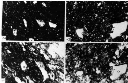
Plate 1 N-1. 須惠器 (大塚) 出土地: 江釣子村猫谷地 1: 石英, 斜長石, 火山ガラスおよびチャートがみられる。(平行ニコル) 2: 同上。(偏光ニコル) 3: 滑結晶を示す石英および斜長石。(平行ニコル) 4: 同上。(偏光ニコル)
