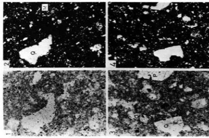
Plate 3 N-3. 須惠器 (坏) 出土地: 江釣子村猫谷地 1, 3: 石英, 長石, 角閃石, 輝石などの結晶片とチャート, 斑鉄質火山岩などの岩片より構成される。(平行ニコル) 2, 4: 同上。(偏光ニコル)
