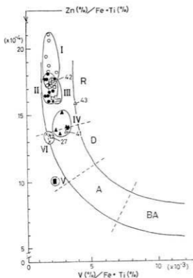
第2図 強磁性鉱物のV-Znベルトと粉状バミスの岩質の関係
