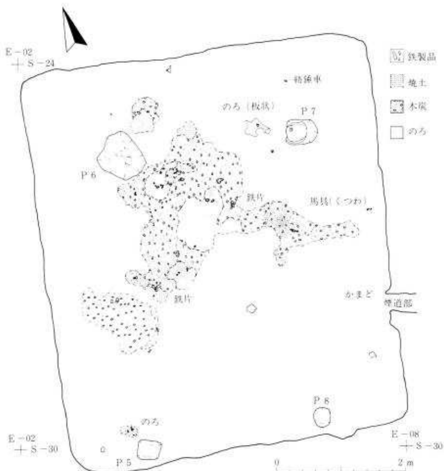
(第11図) C150住居跡鉄器、のろ等出土状況図
