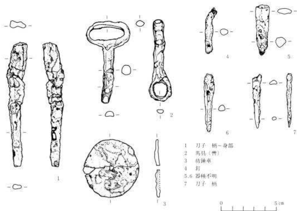
(第10図) C150住居跡出土、鉄製品実測図
