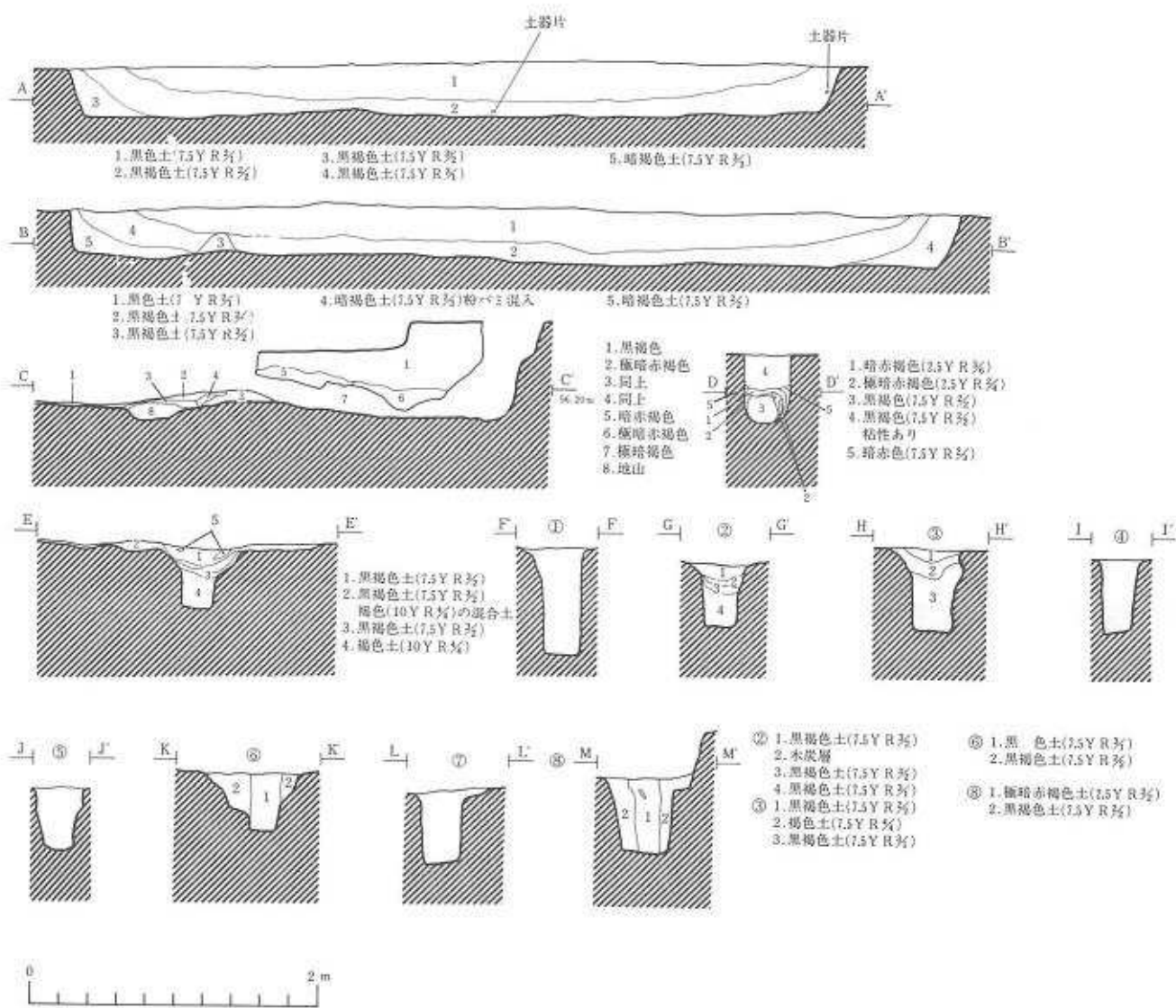
(第5图) C150住居跡平断面图
