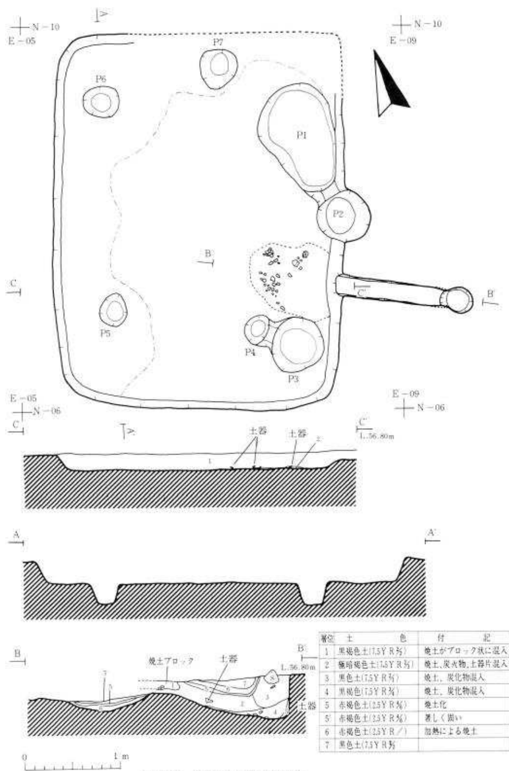
(第3図) BG 53住居跡平断面図
