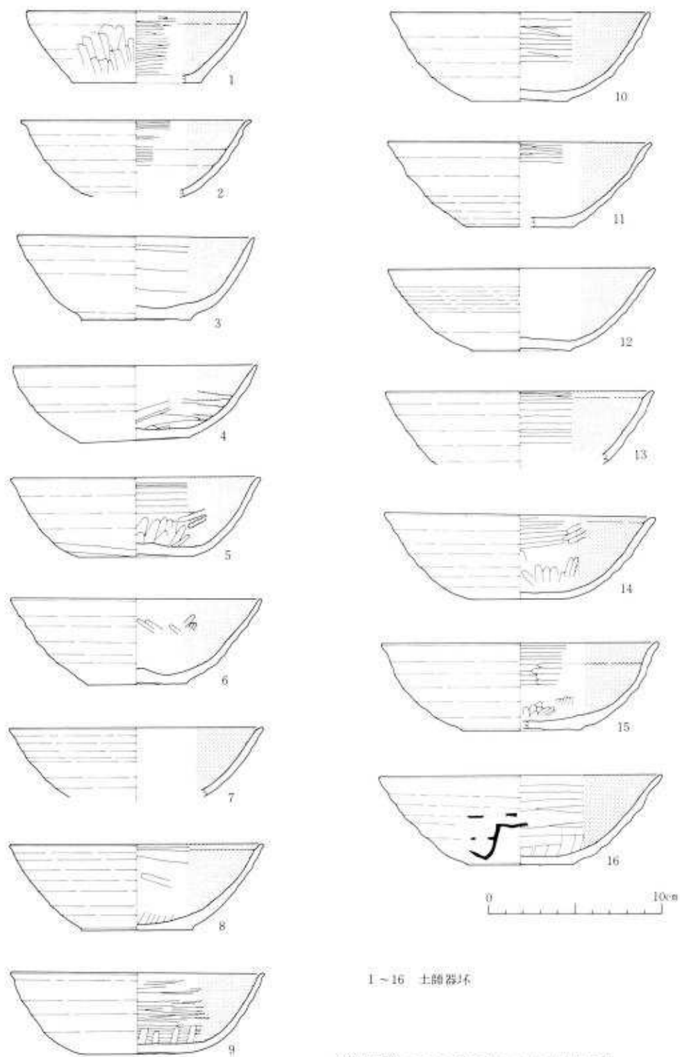
(第15图) C E 36住居跡出土土器実测图
