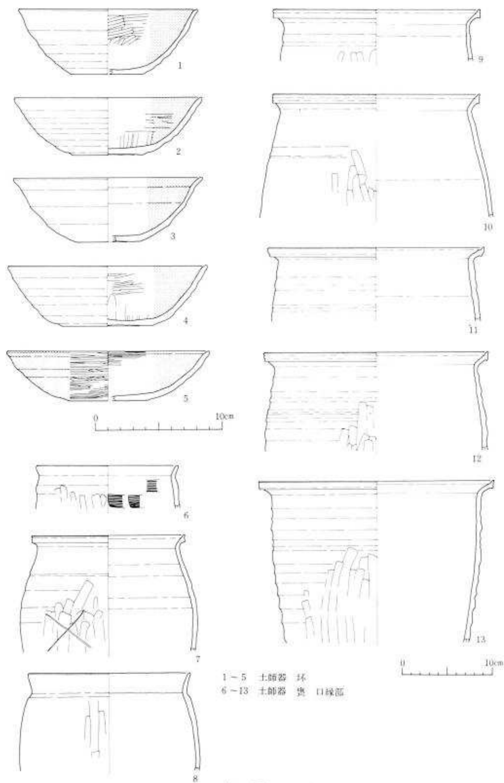
(第6图) C150住居跡出土土器実測图
