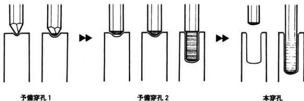
第112図 穿孔工程 手法復元模式図
