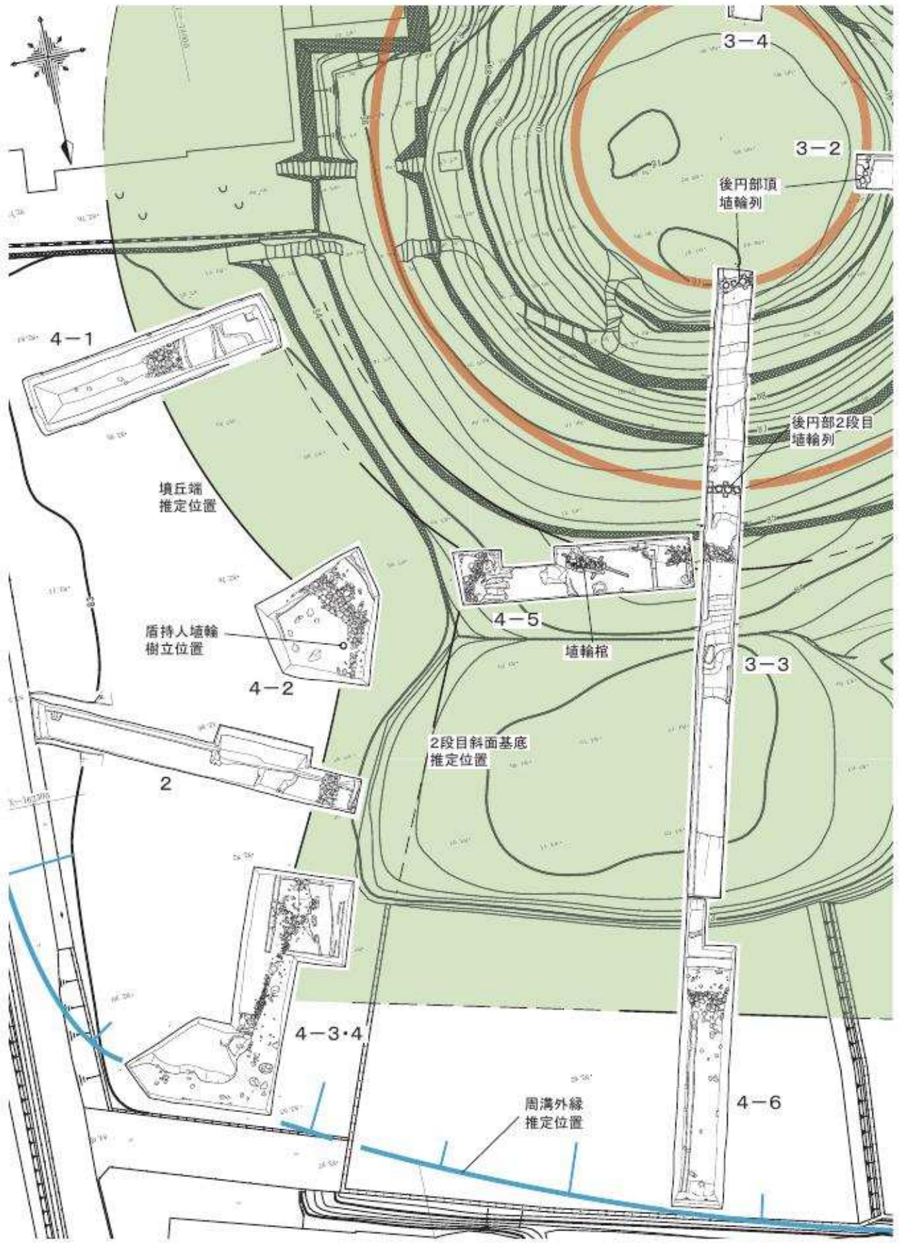
図13 埴丘北東側のトレンチ配置図 (S = 1/300)
