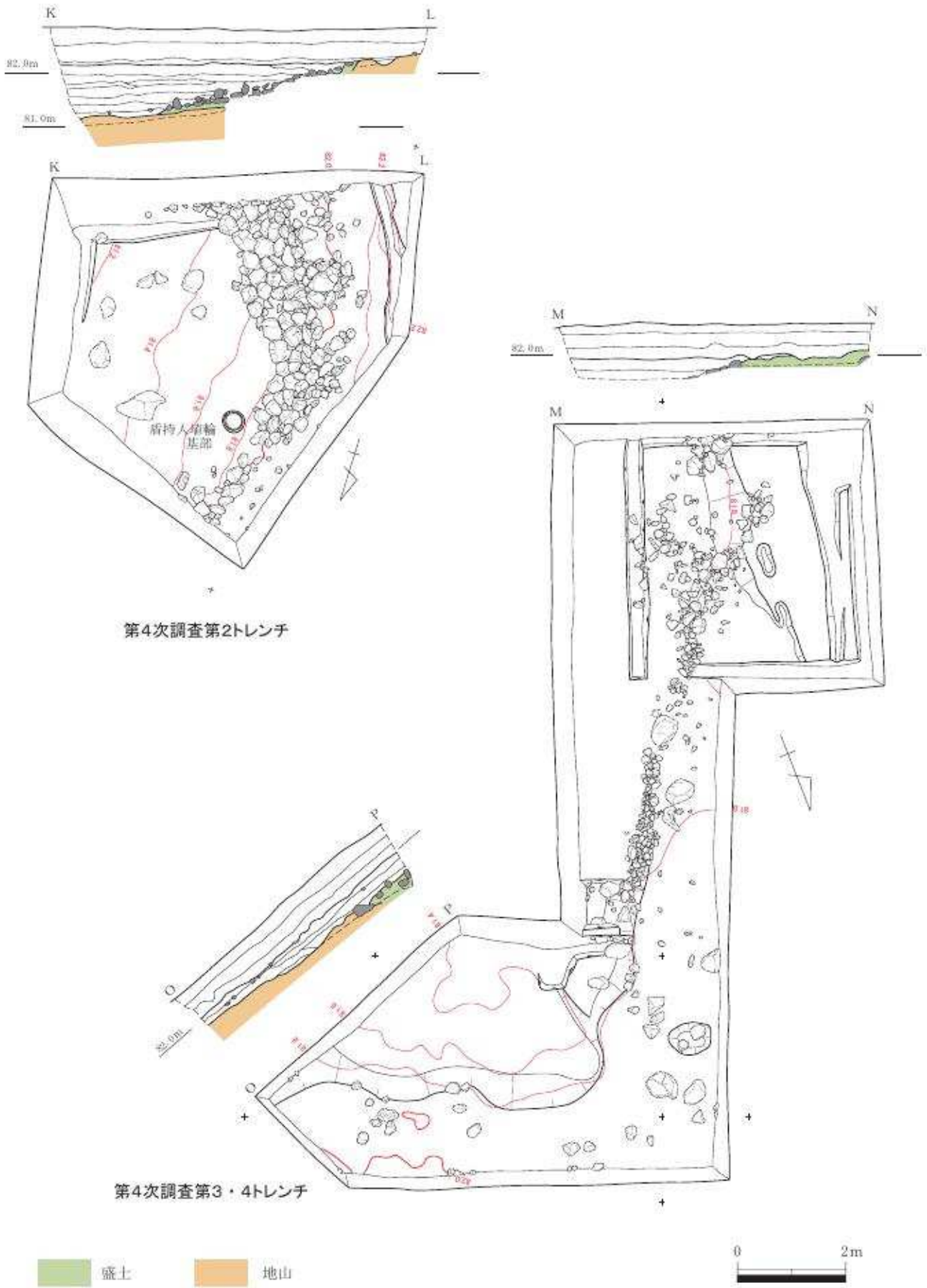
図8 墳丘東側のトレンチ平面・断面図② (S = 1/100)
